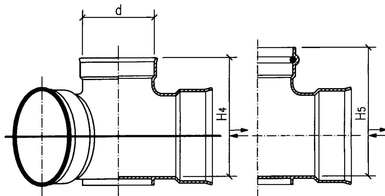
d型立、剖面图
