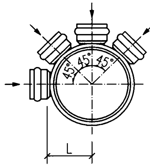
b型平面图 (四)
