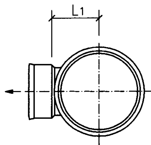
b型平面图
