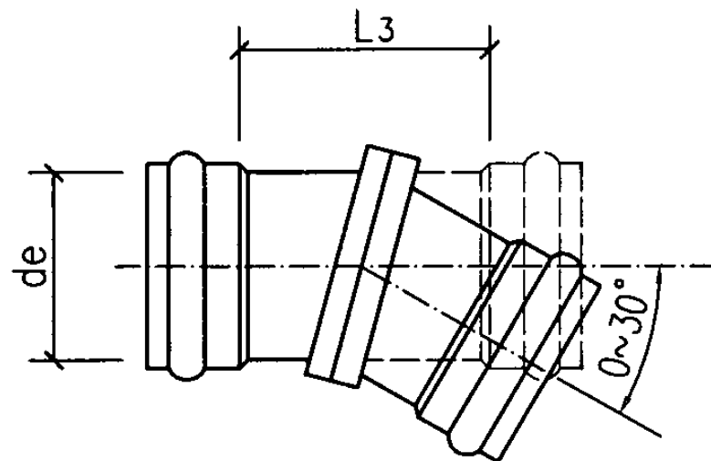
c型可变角接头
