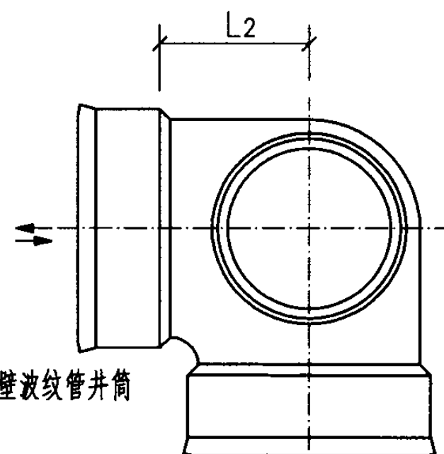
c型立、剖面图
