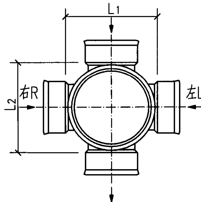
b型平面图
