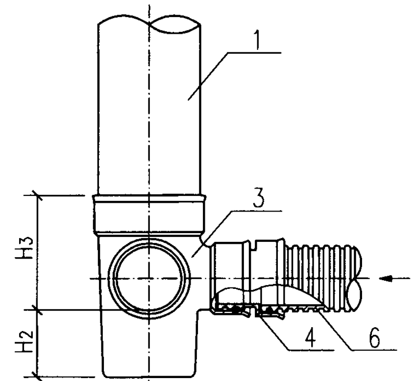
B型立面图
