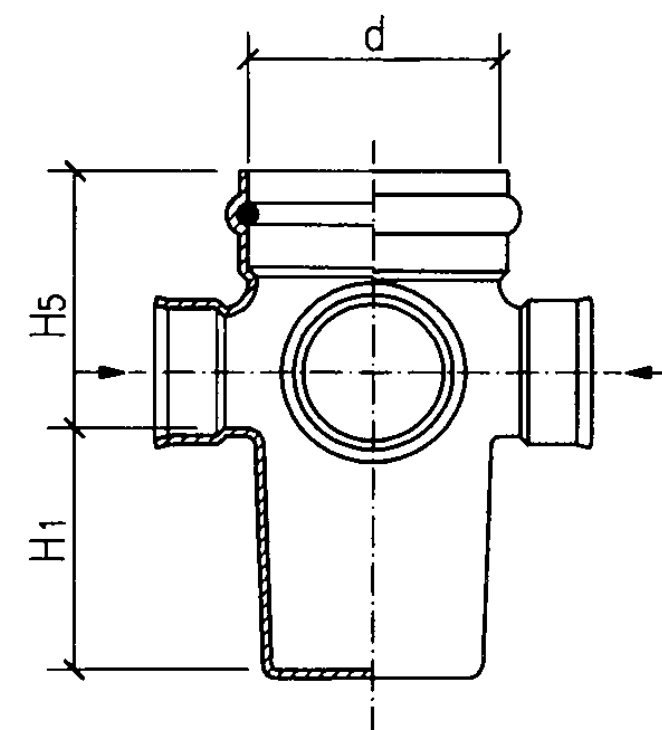
d型立、剖面图
