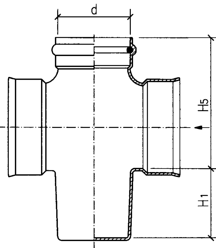
d型立、剖面图
