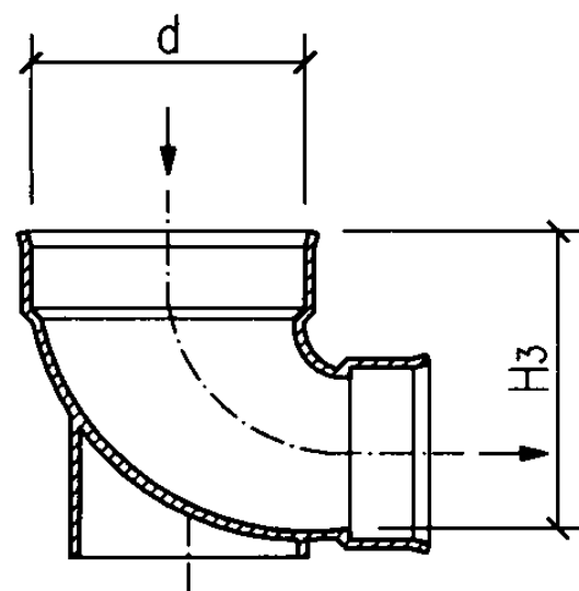
c型剖面图
