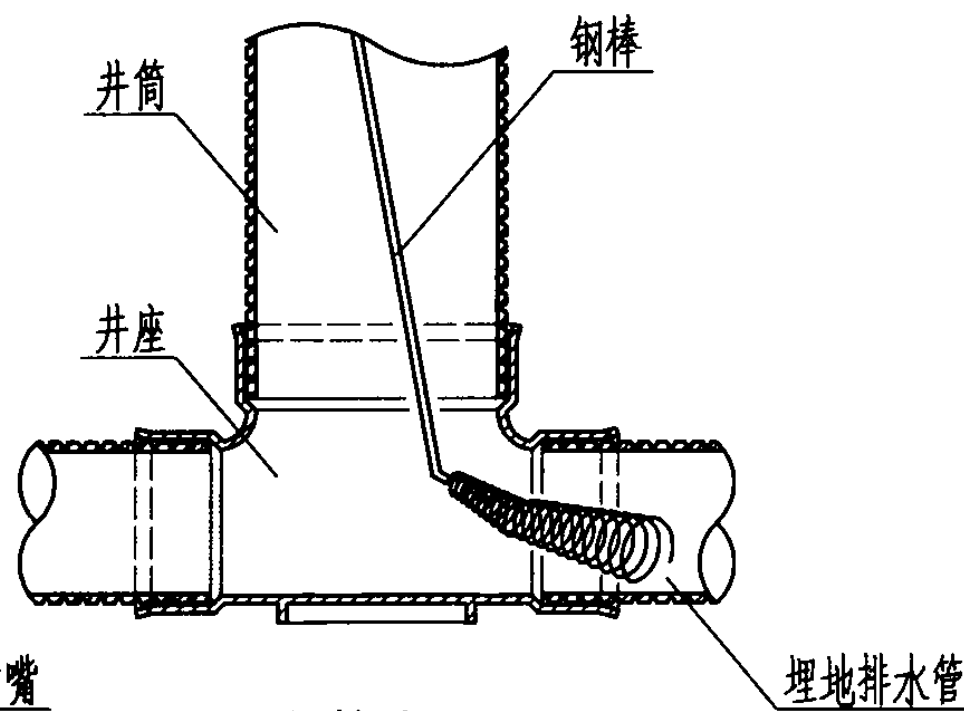
钢棒疏通
