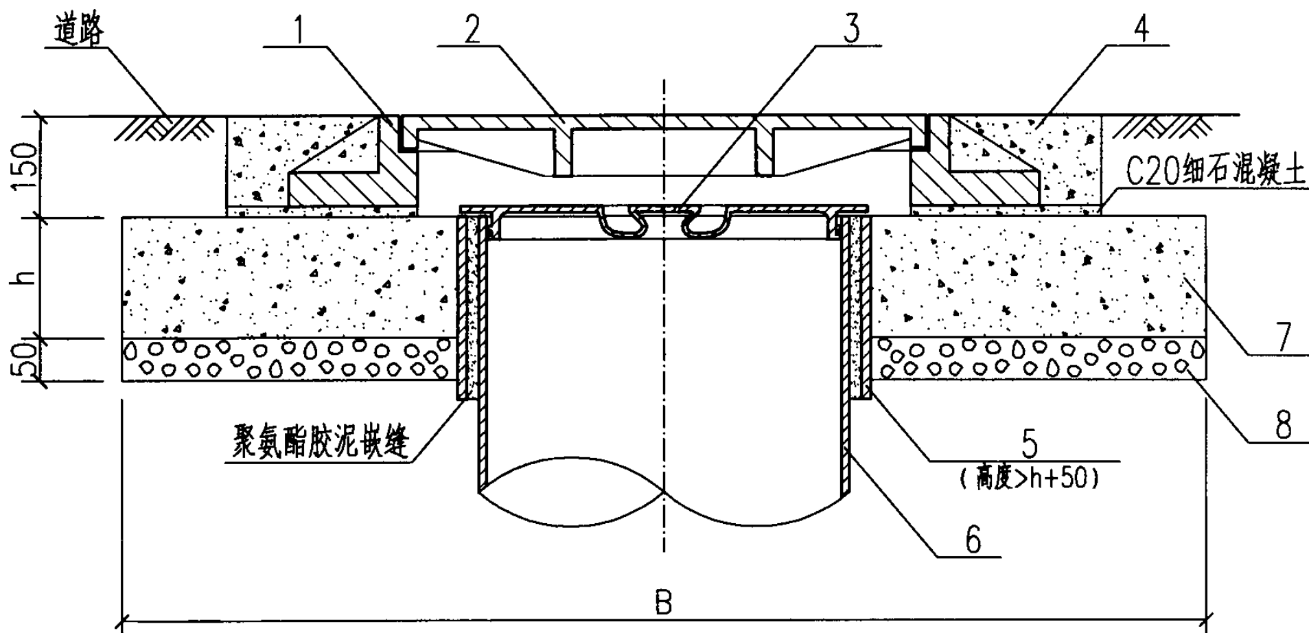
防护盖座基础结构图
