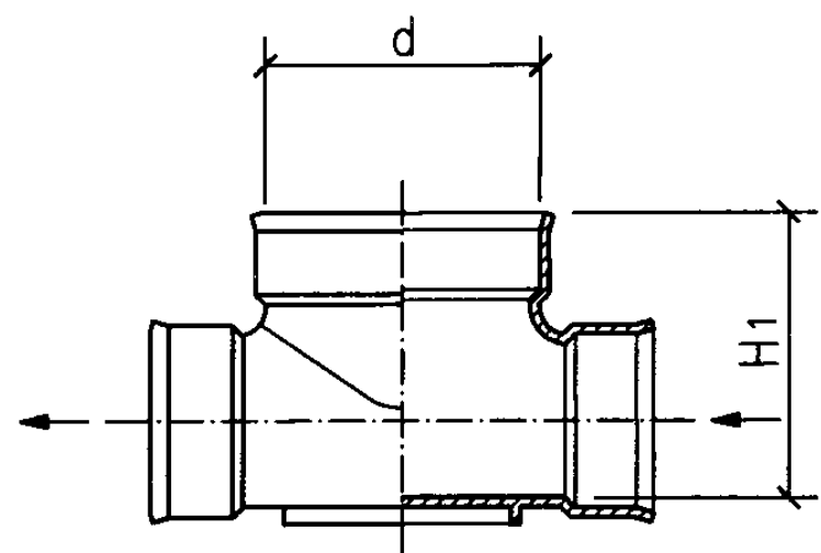
a型立、剖面图
