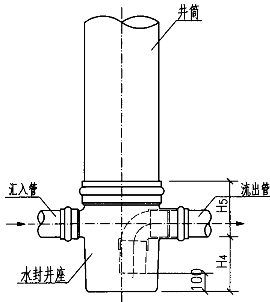
立面图
