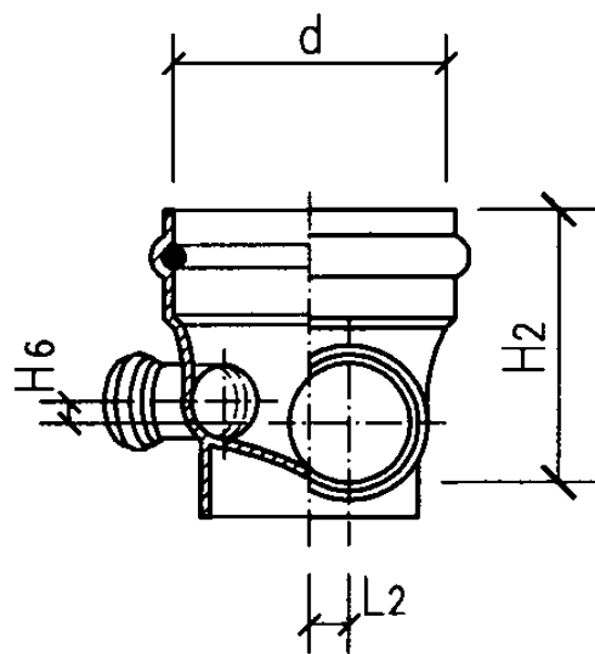
b型立、剖面图
