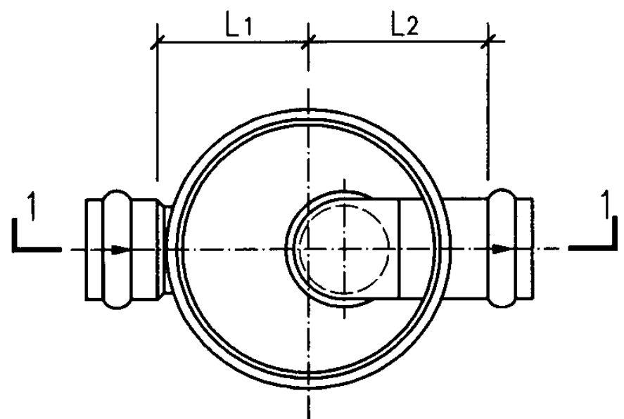
a型平面图
