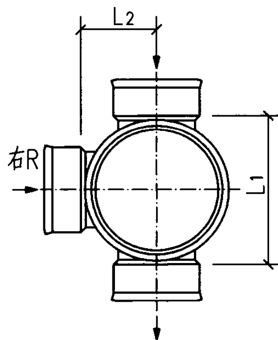
b型平面图
