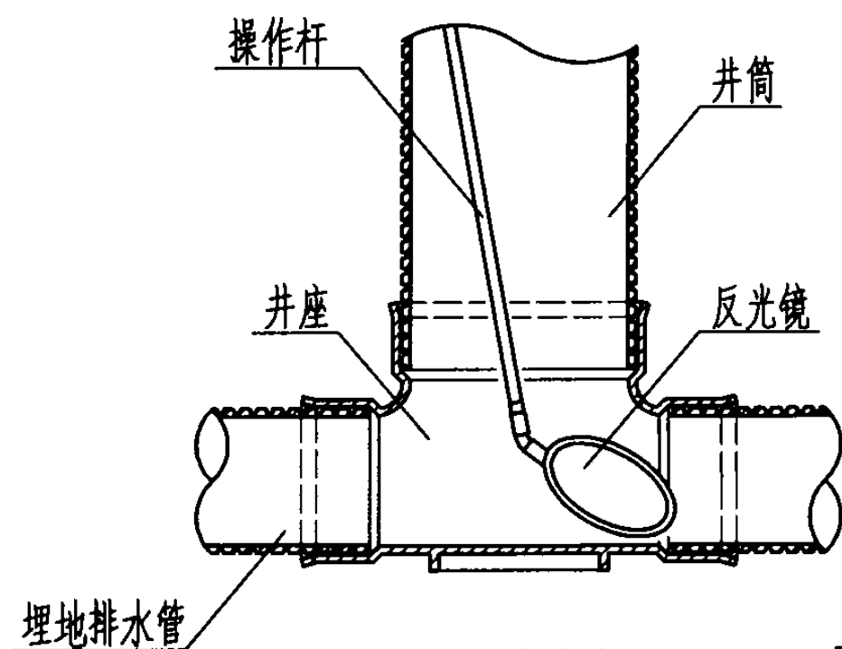
反光镜检查
