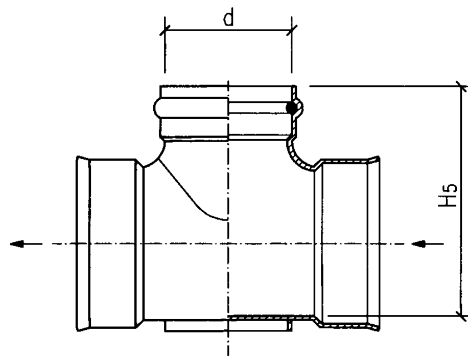
e型立、剖面图
