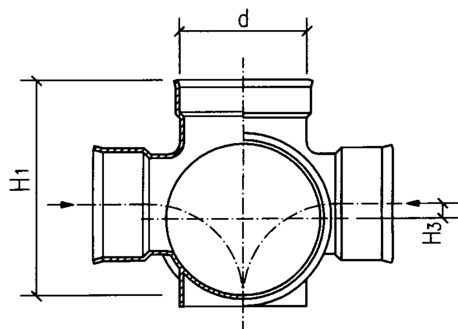
c型立、剖面图
