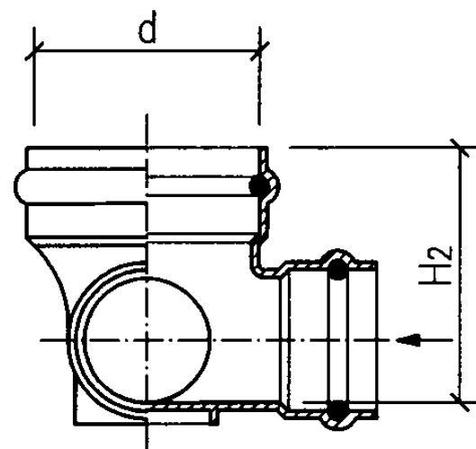
b型立、剖面图
