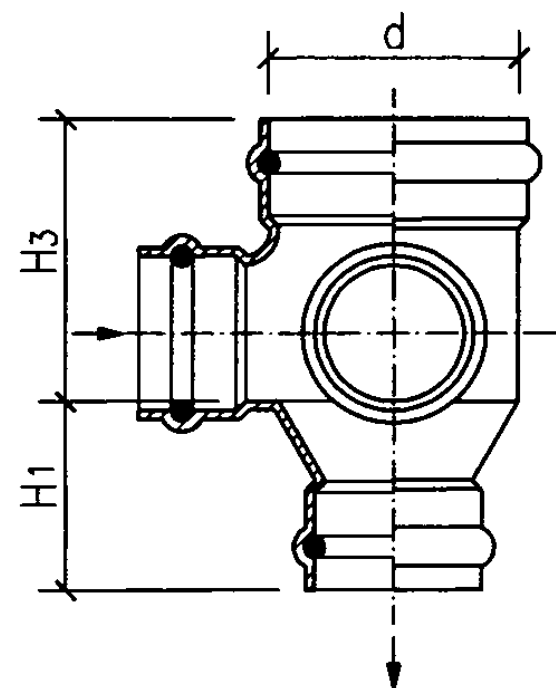
b型立、剖面图
