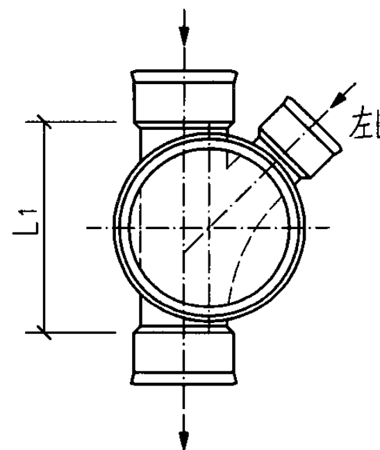
c型平面图
