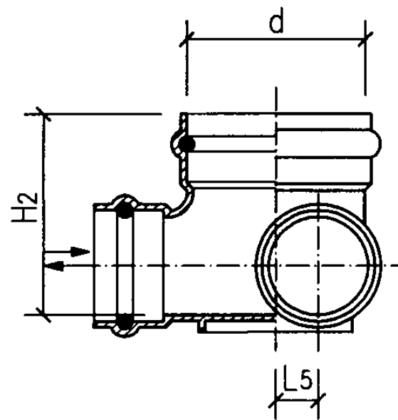
b型立、剖面图
