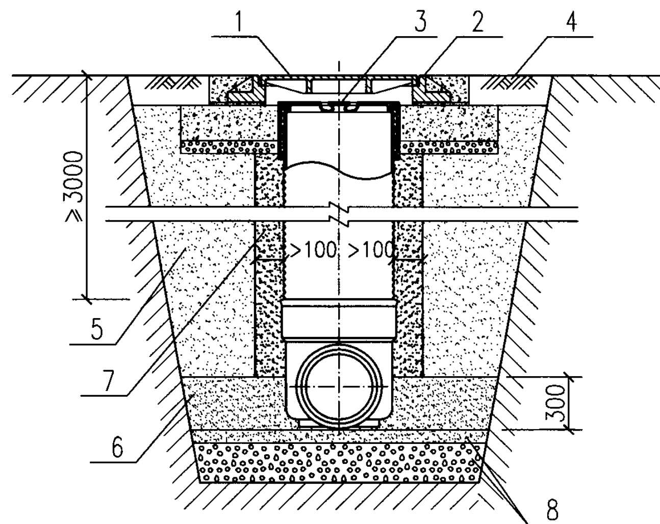
减少下曳力处理回填
