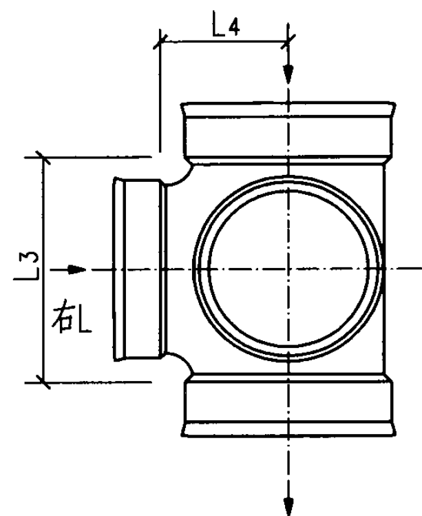
e型平面图
