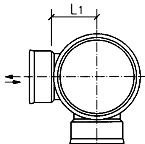
b型立、剖面图
