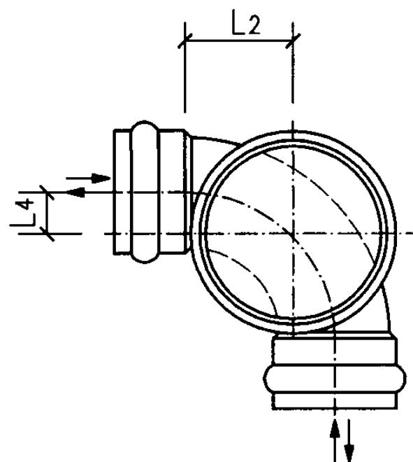
b型平面图
