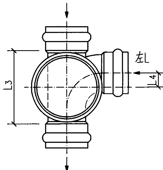
b型平面图
