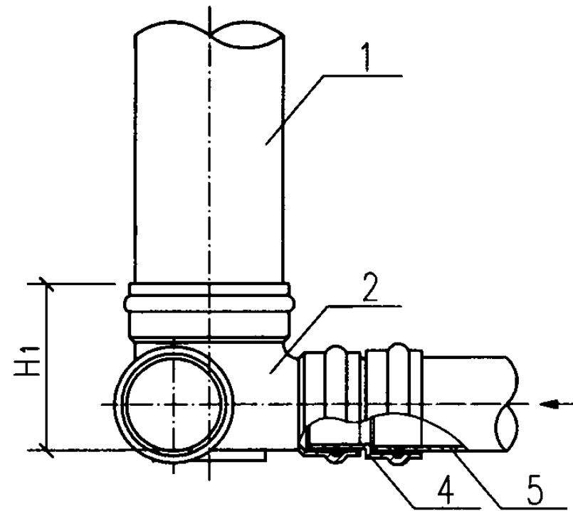
A型立面图
