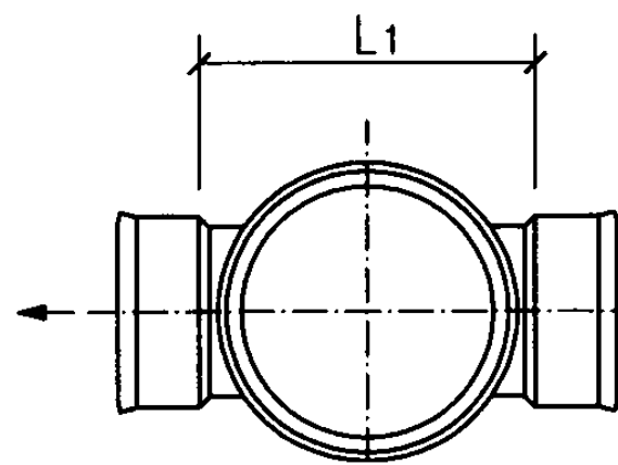
a型平面图
