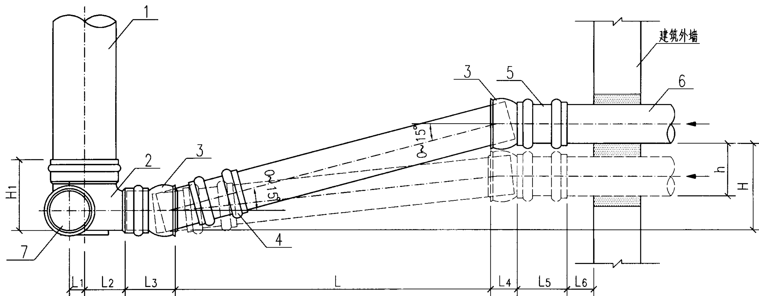
调整坡度立面图
