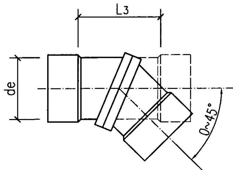
a型可变角接头
