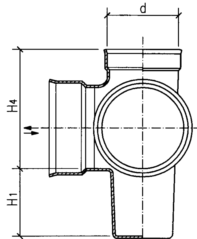
c型立、剖面图
