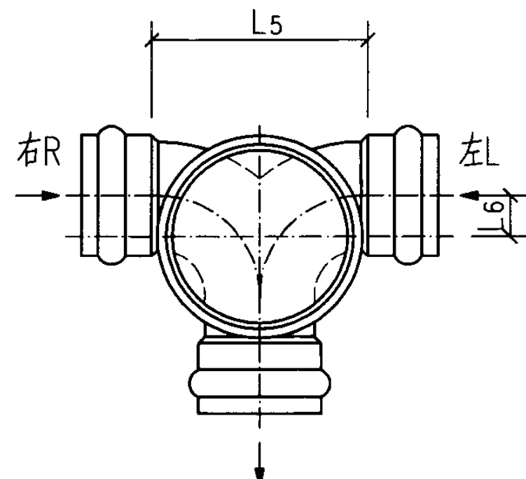
c型平面图
