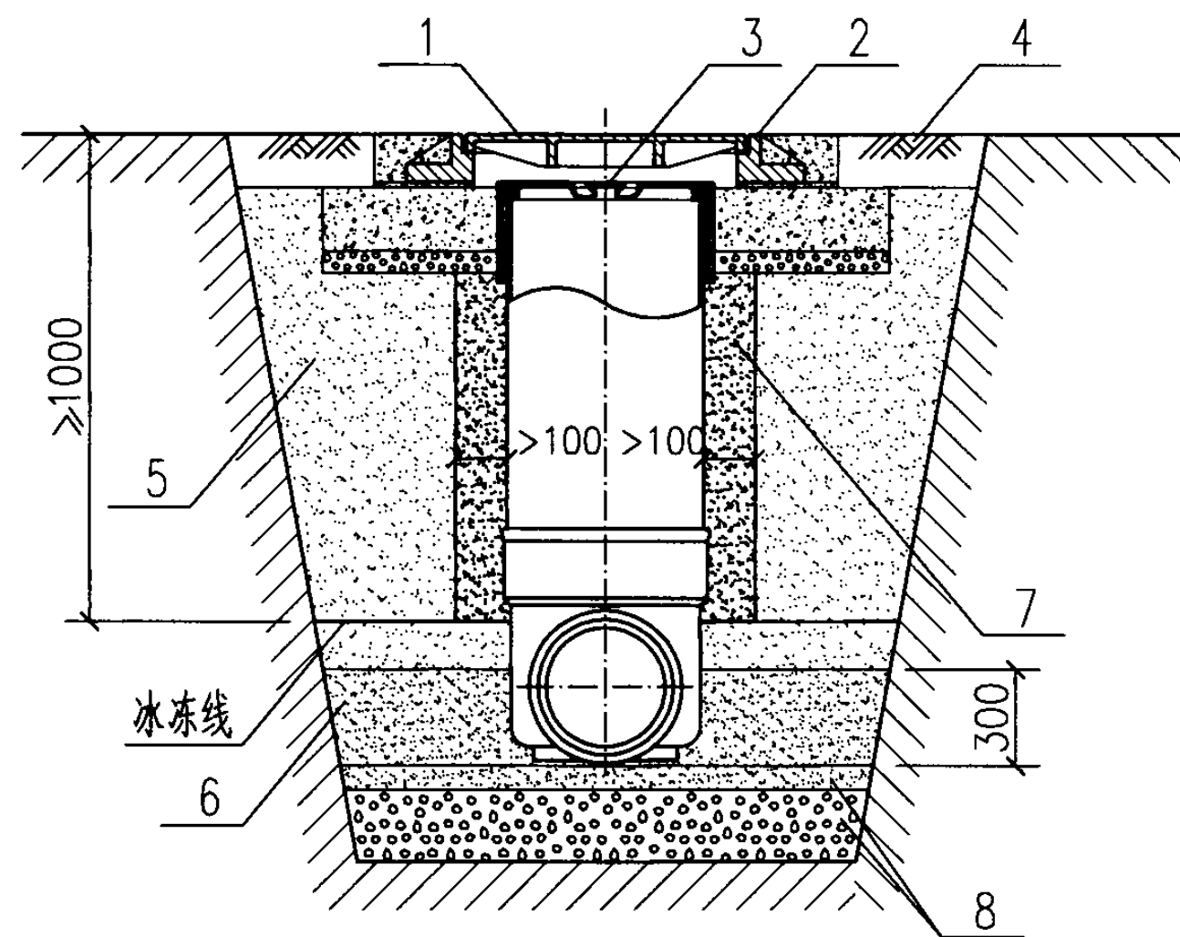
防冻处理回填 (防护井盖)
