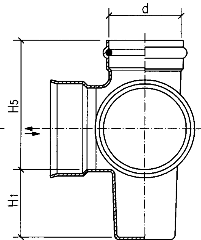
d型立、剖面图
