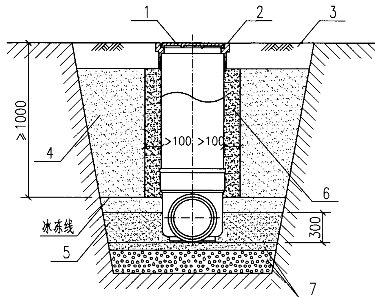
防冻处理回填 (非防护井盖)
