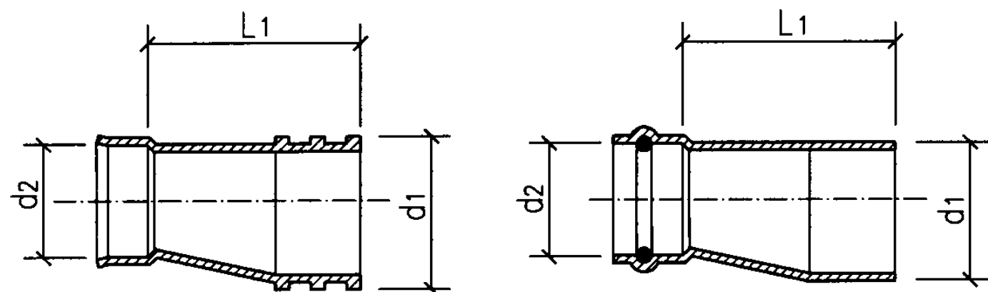
偏心渐扩异径接头
