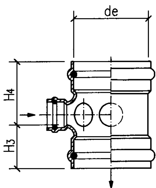
b型立、剖面图 (三)
