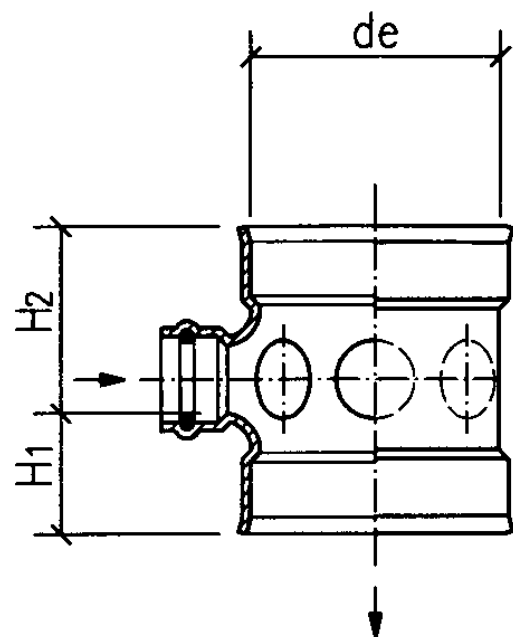
a型立、剖面图 (四)
