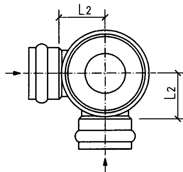
b型平面图
