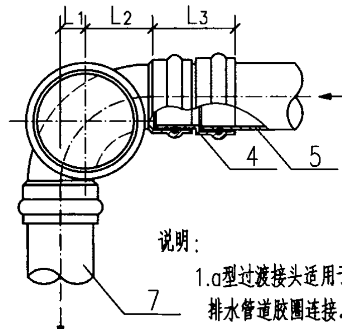
A型平面图
