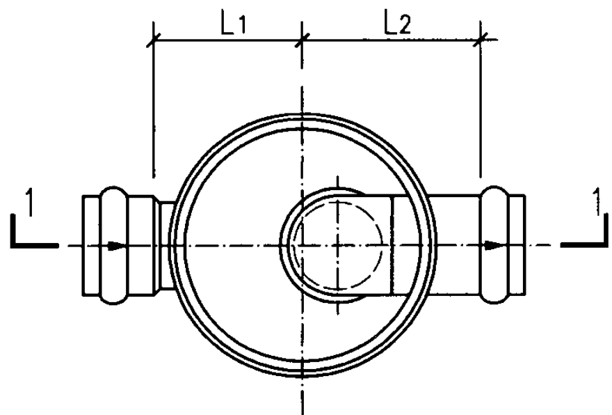
b型平面图
