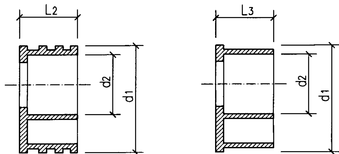
偏心异径接头
