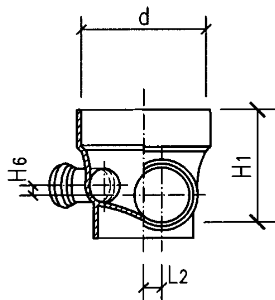
a型立、剖面图
