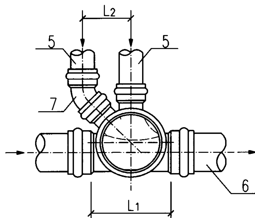
A型平面图
