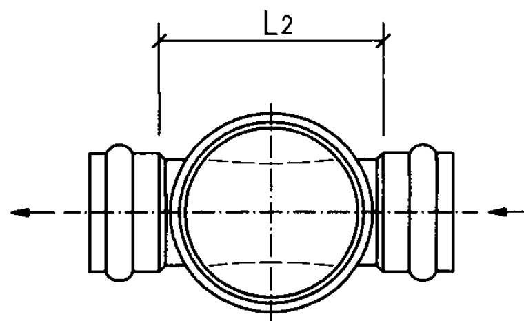
b型平面图
