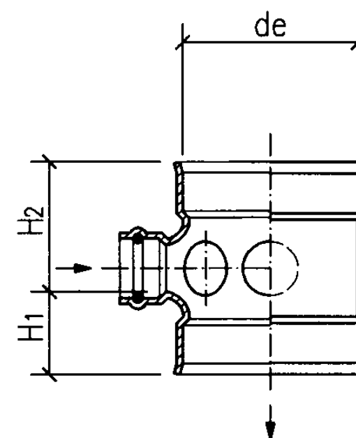
a型立、剖面图 (三)
