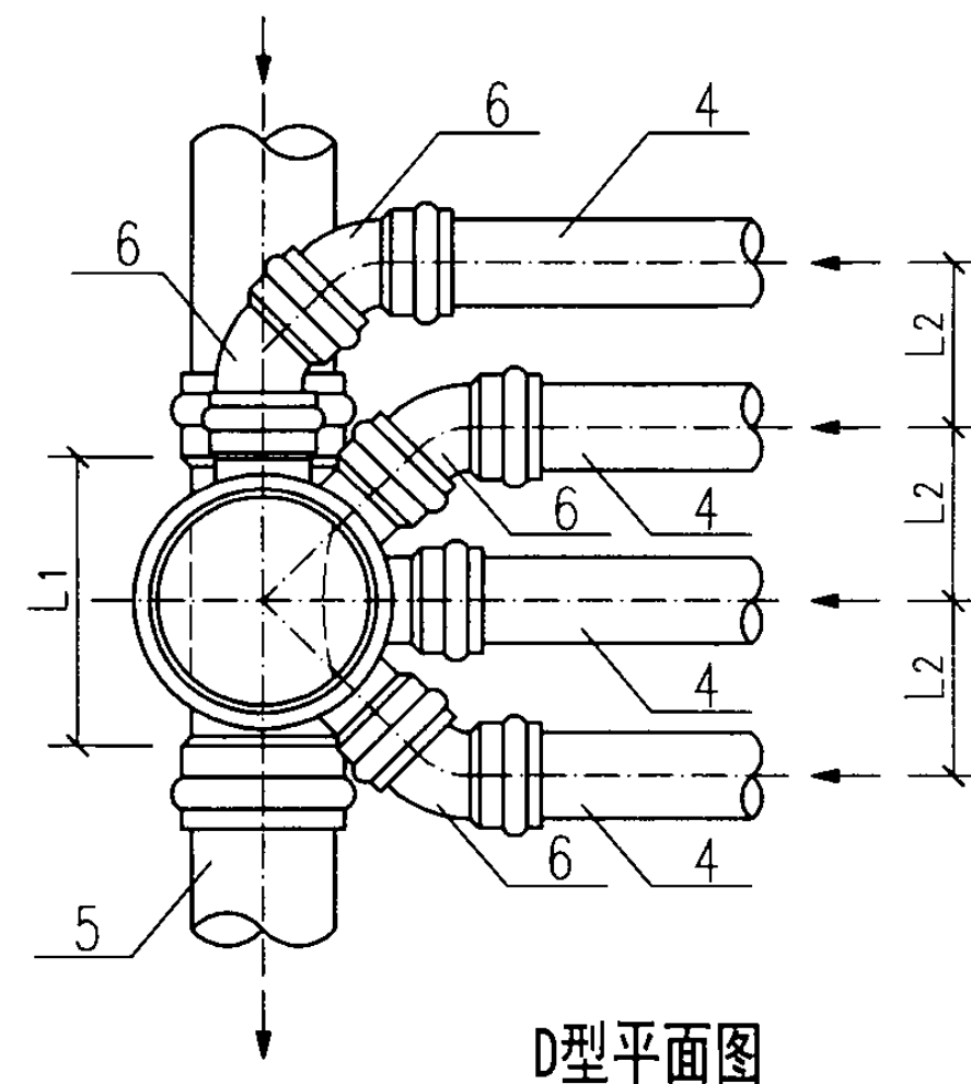
多根排出管连接 (3~4根)
