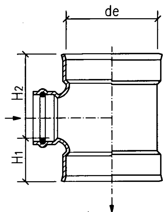
a型立、剖面图 (一)
