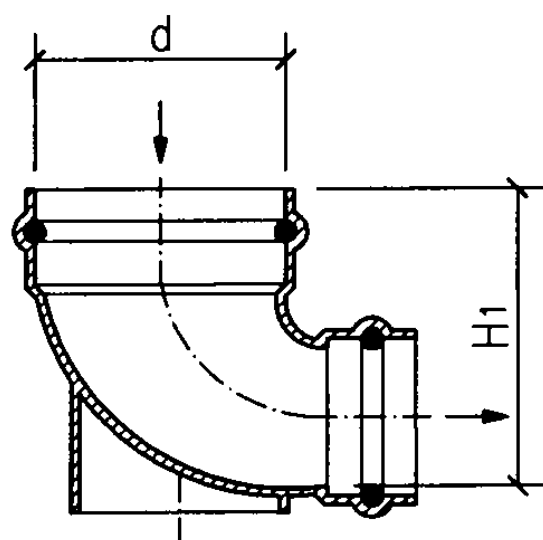
a型剖面图
