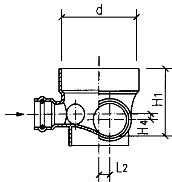
a型立、剖面图
