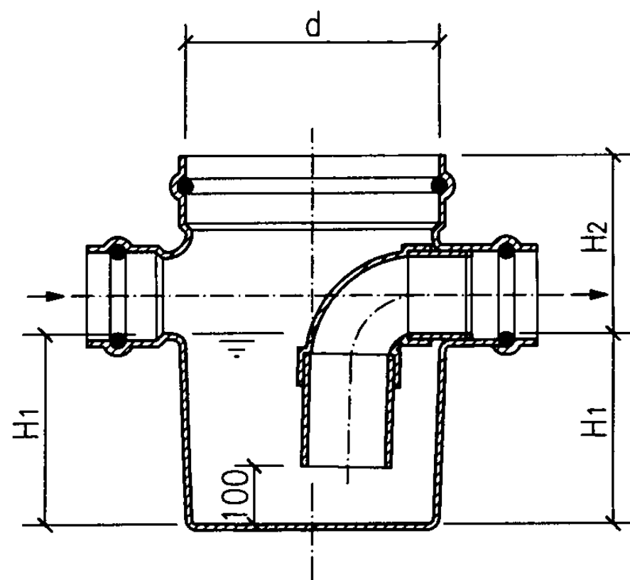
a型1-1
