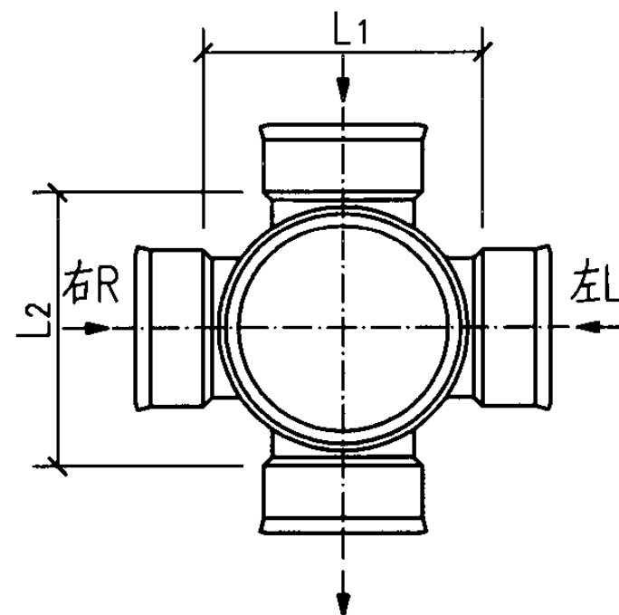
a型平面图
