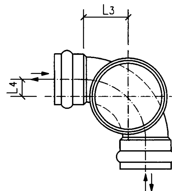
c型平面图
