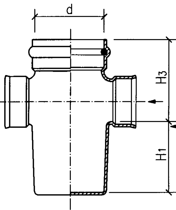
b型立、剖面图
