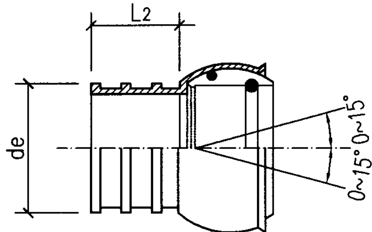
b型球形接头
