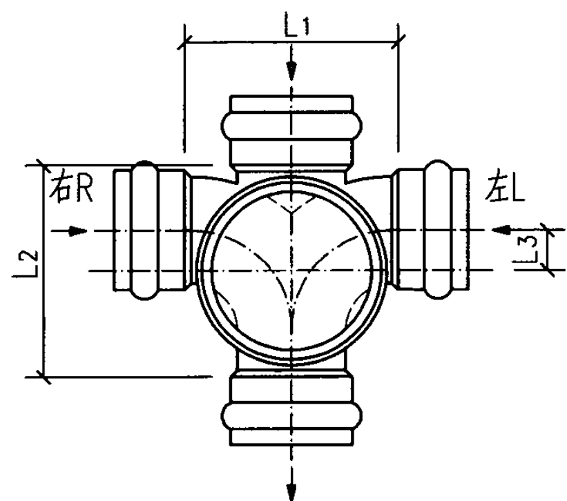
a型平面图
