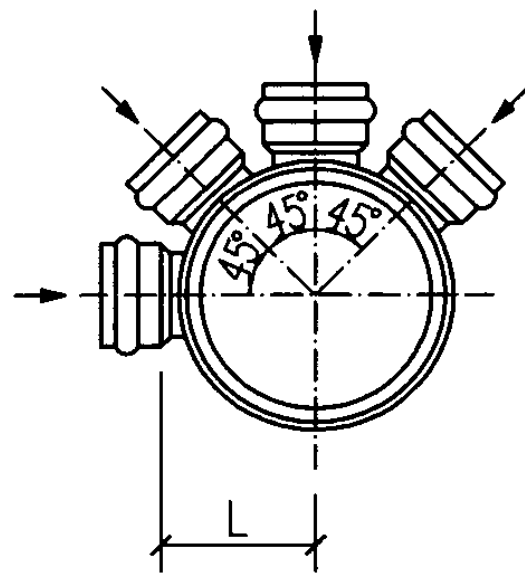
a型平面图 (四)
