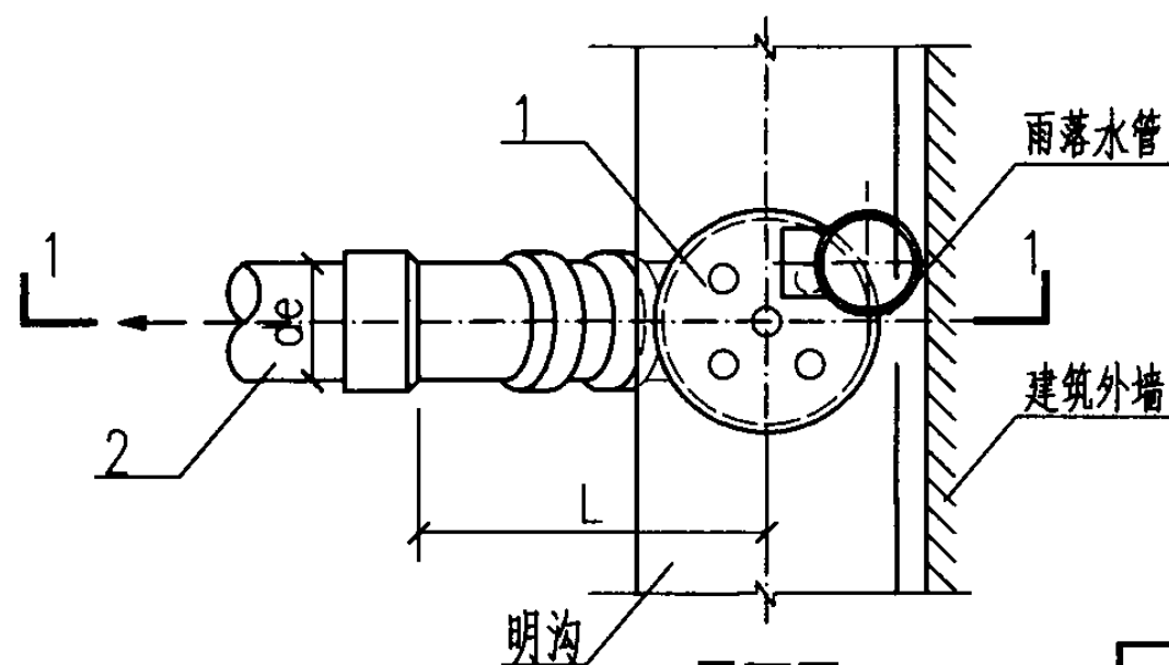
平面图
