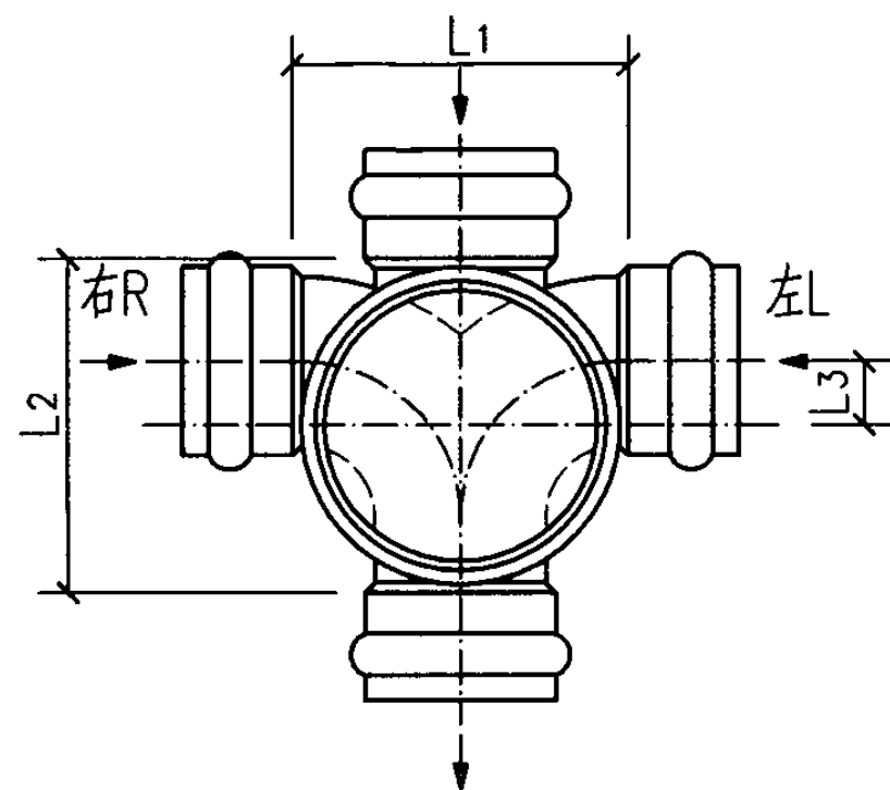
b型平面图
