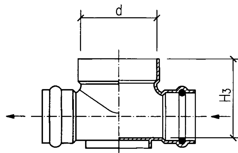
c型立、剖面图
