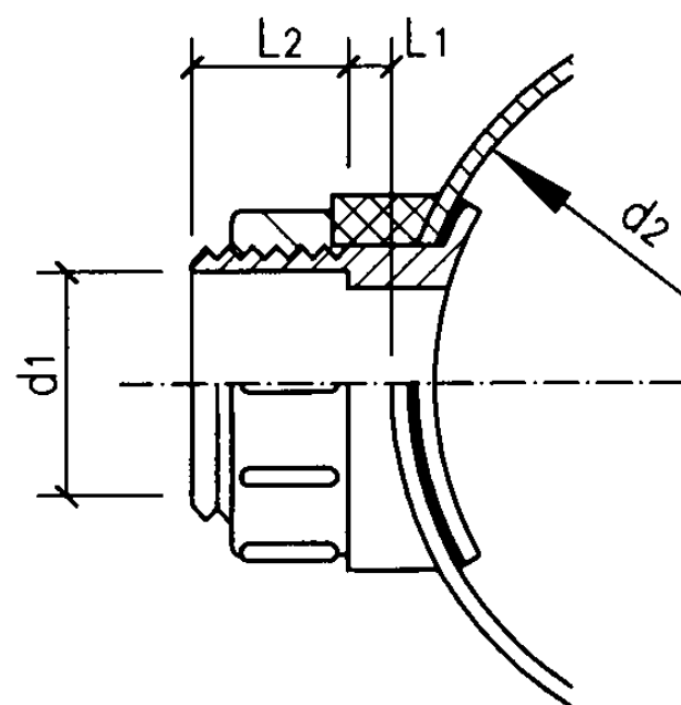
附加接头
