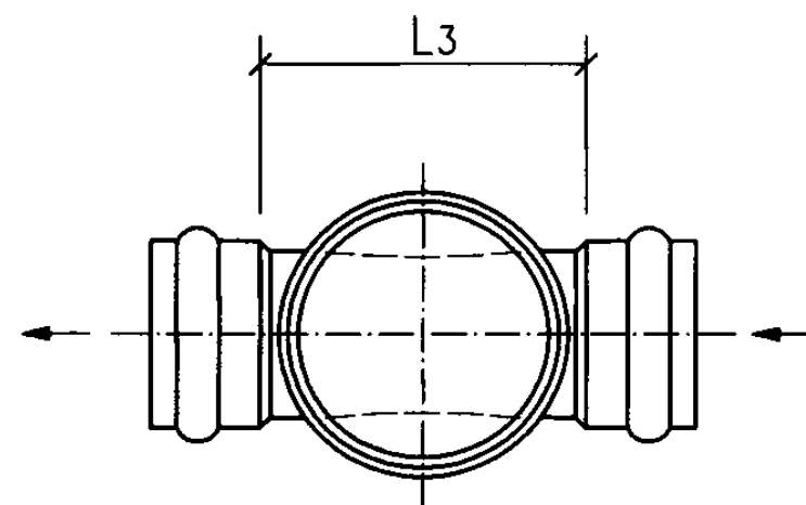
c型平面图
