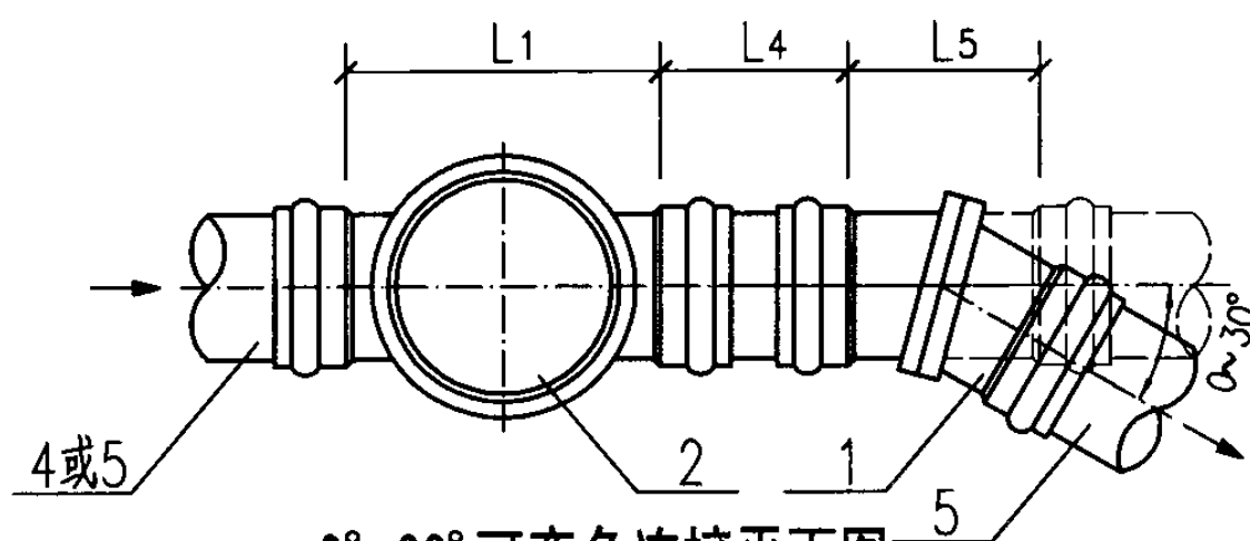
0°~30° 可变角连接平面图
