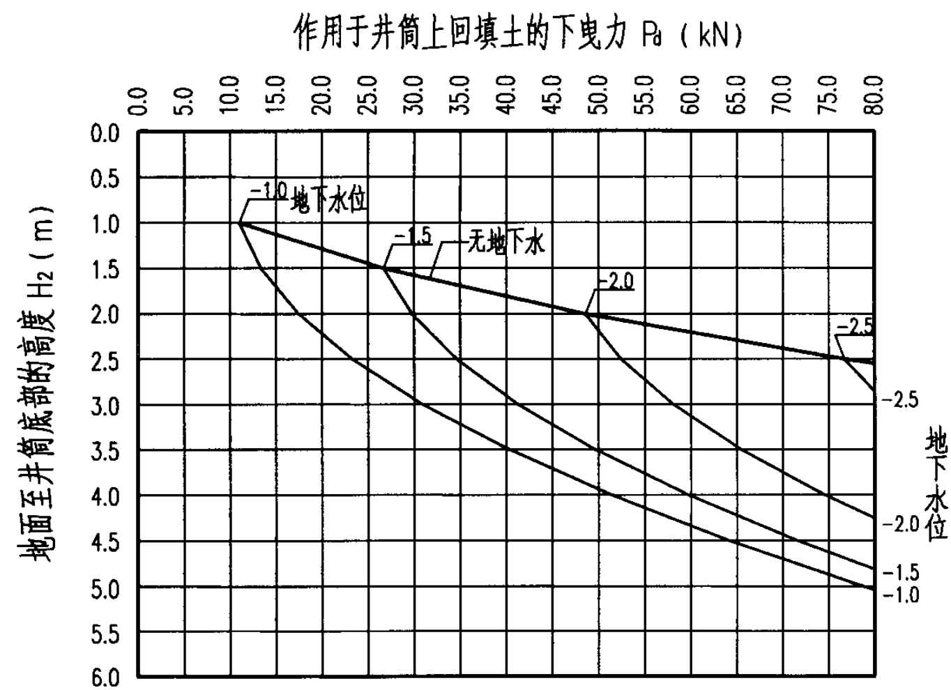
de630井筒回填土下曳力图(软土土质)
