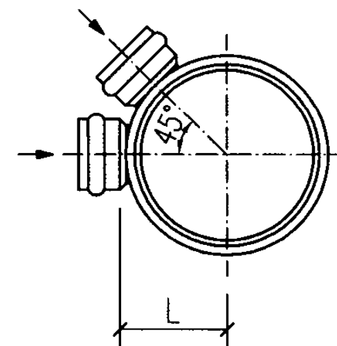
b型平面图 (二)
