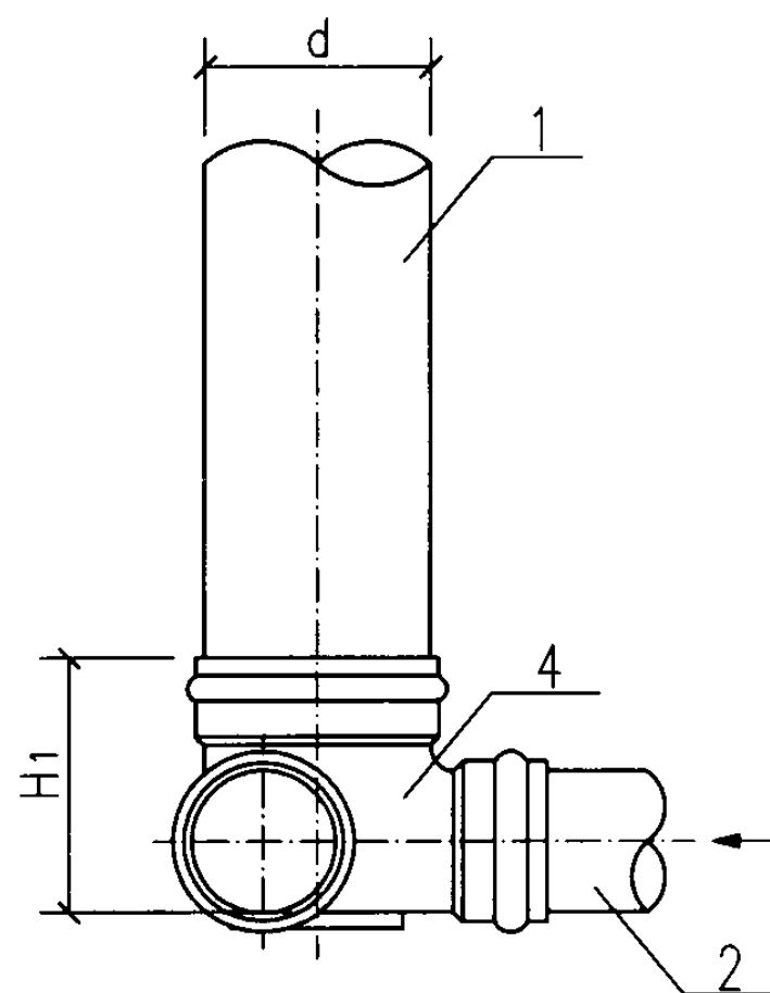
A型立面图
