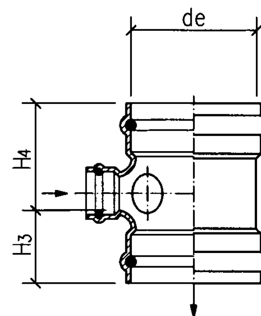
b型立、剖面图 (二)
