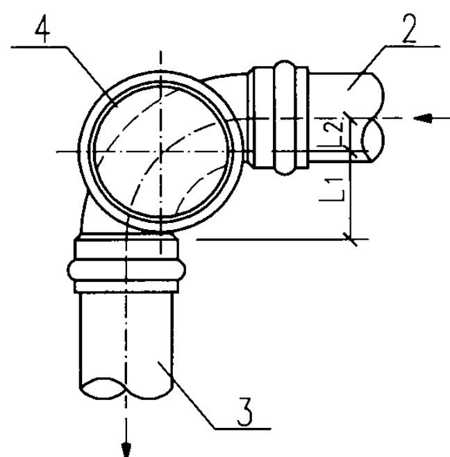
A型平面图
