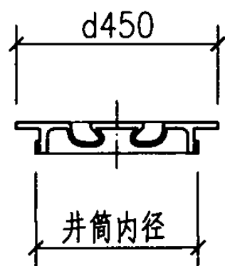
内盖立面图
