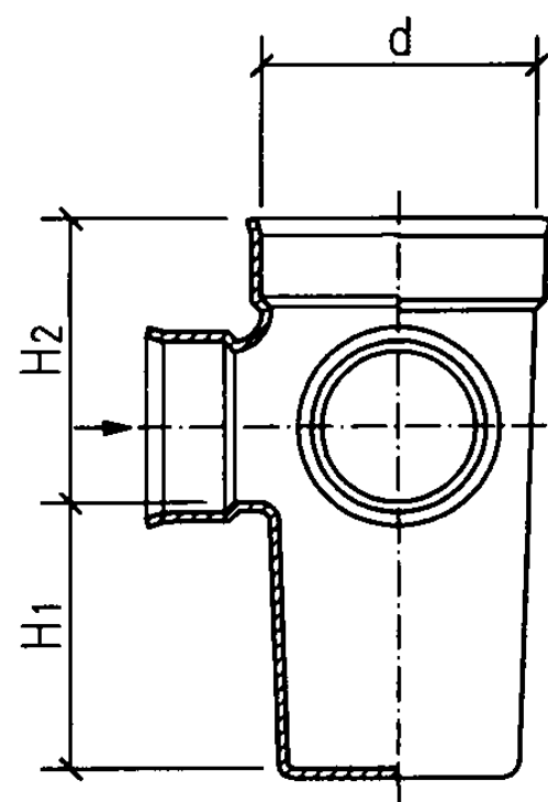
a型立、剖面图
