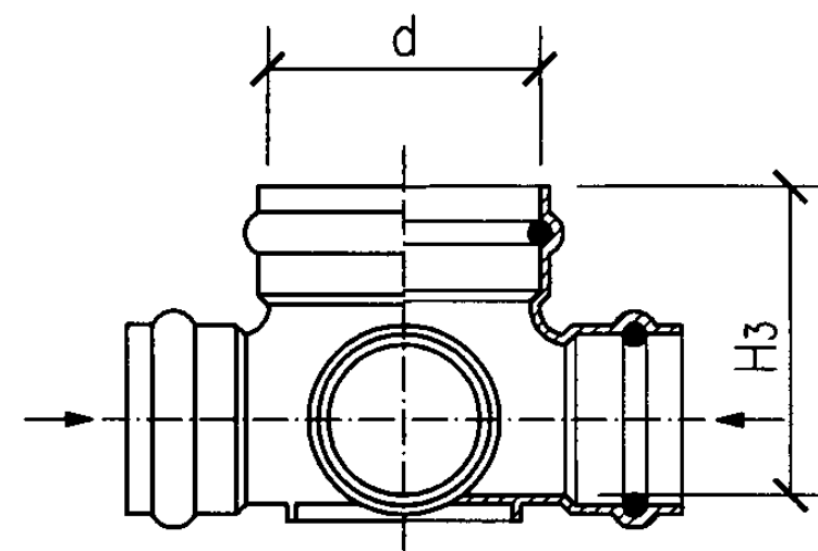
c型立、剖面图
