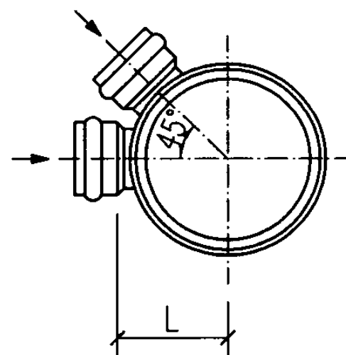
a型平面图 (二)
