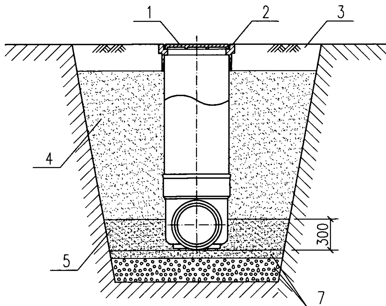
一般回填 (非防护井盖)
