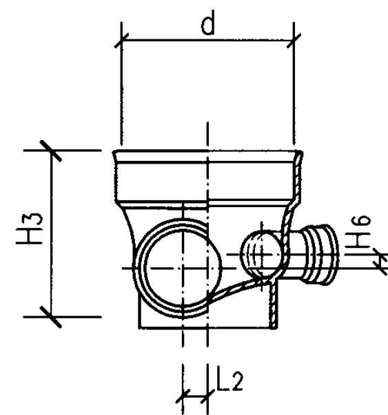
c型立、剖面图
