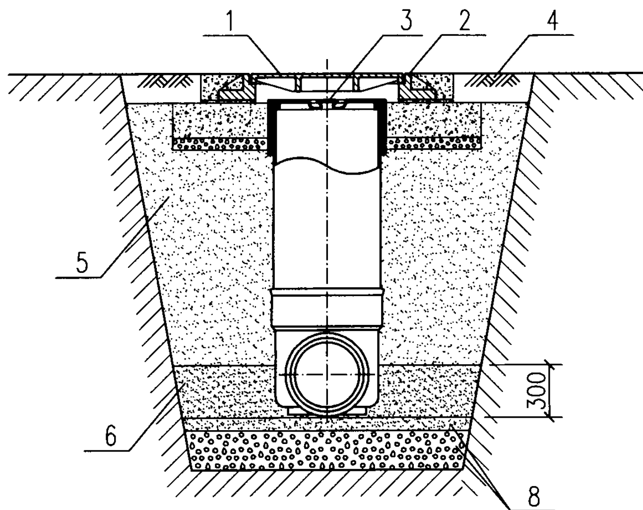
一般回填 (防护井盖)
