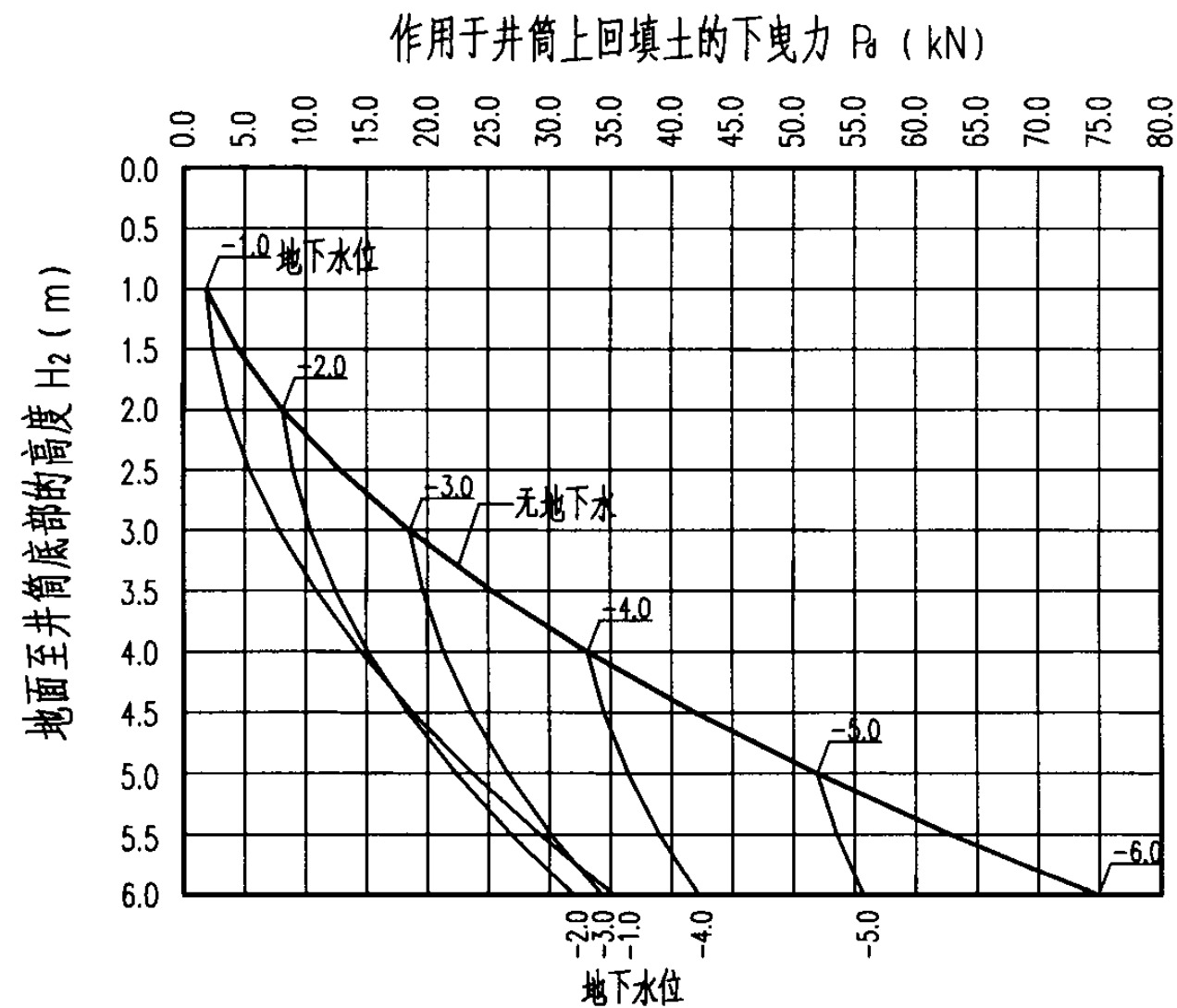
de450井筒回填土下曳力图(砂土土质)
