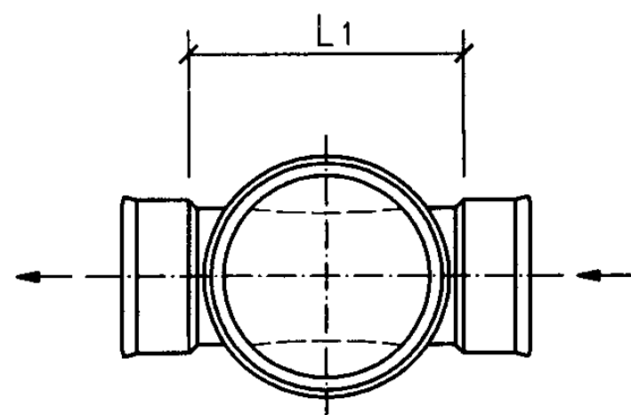
a型平面图
