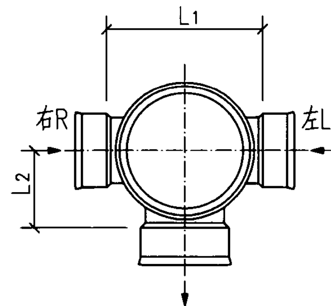
c型平面图
