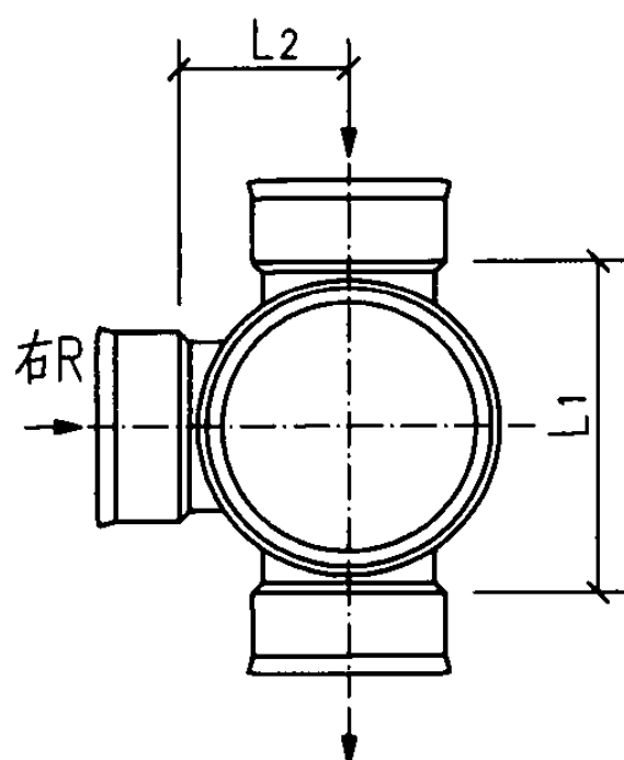
a型平面图
