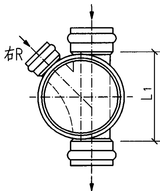
b型平面图
