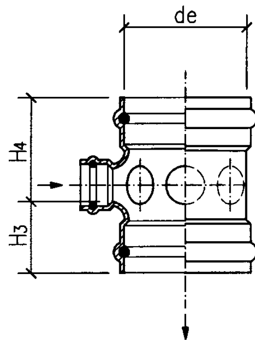
b型立、剖面图 (四)
