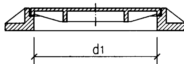
630防护盖座
