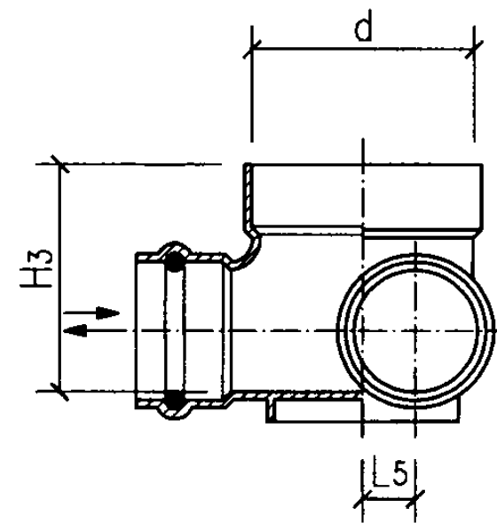
c型立、剖面图
