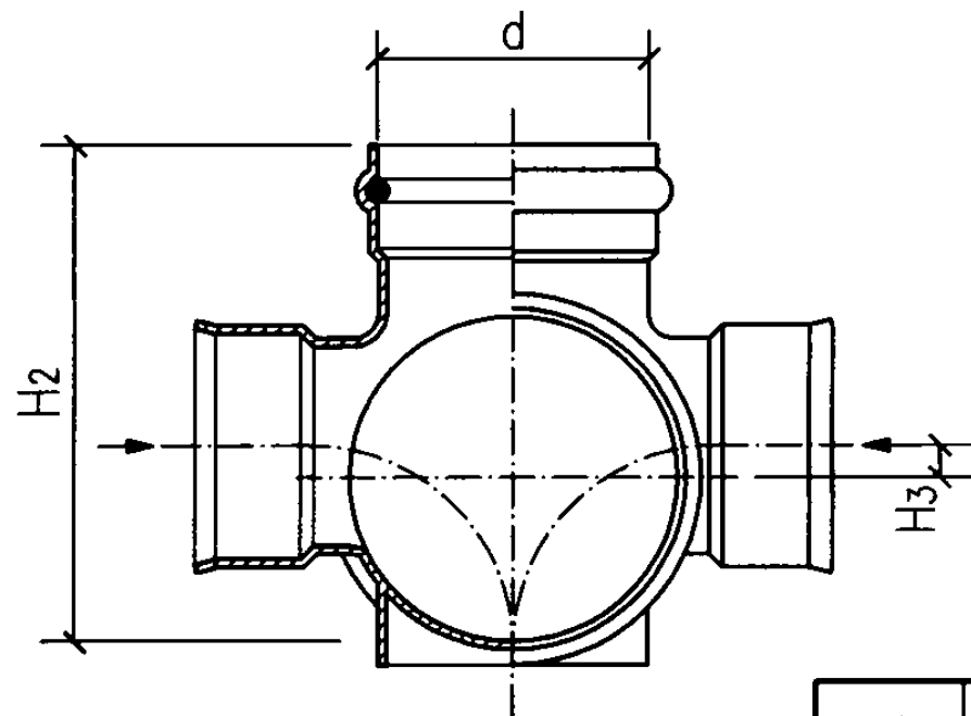
d型立、剖面图
