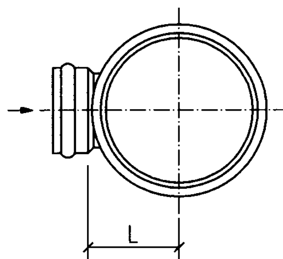
b型平面图 (一)
