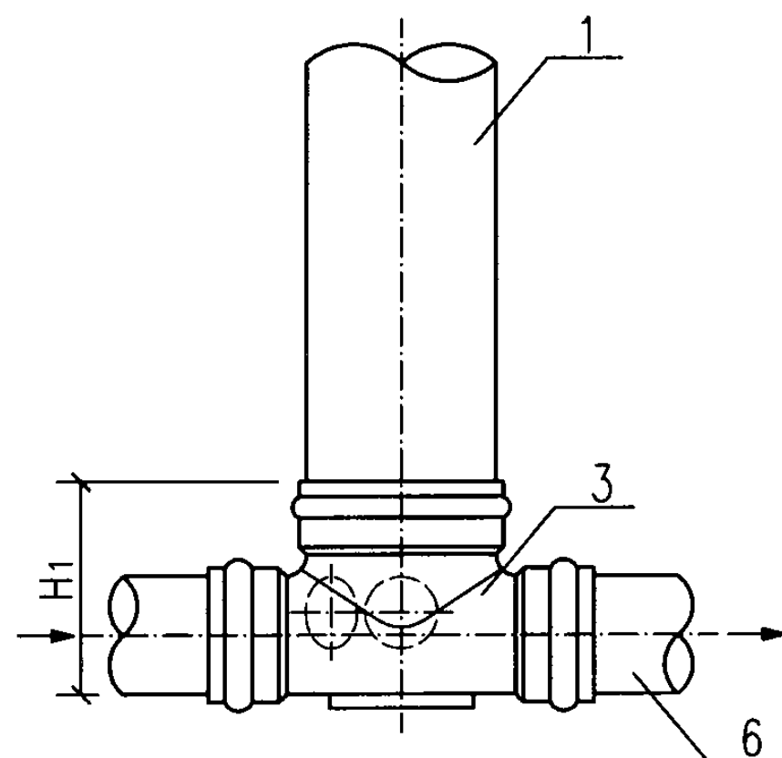
A型立面图
