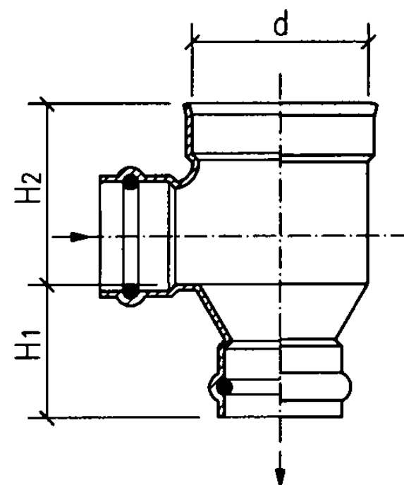
a型立、剖面图
