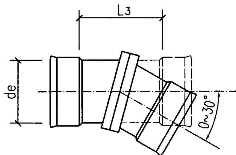
b型可变角接头
