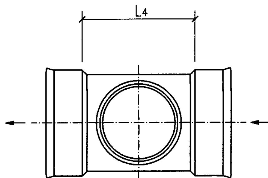
d、e型平面图
