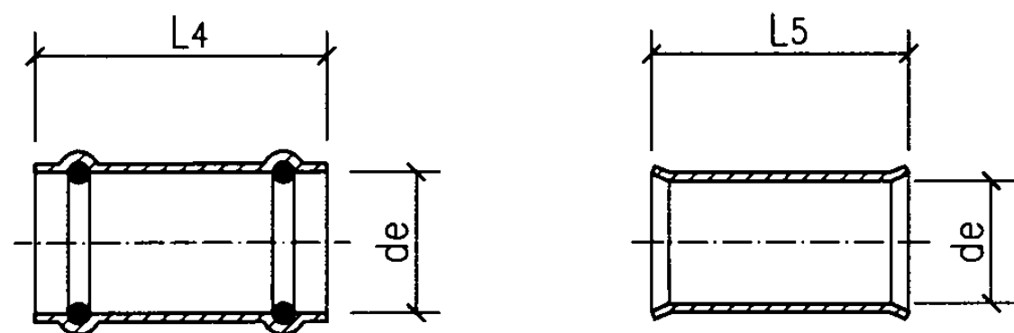
伸缩管接
