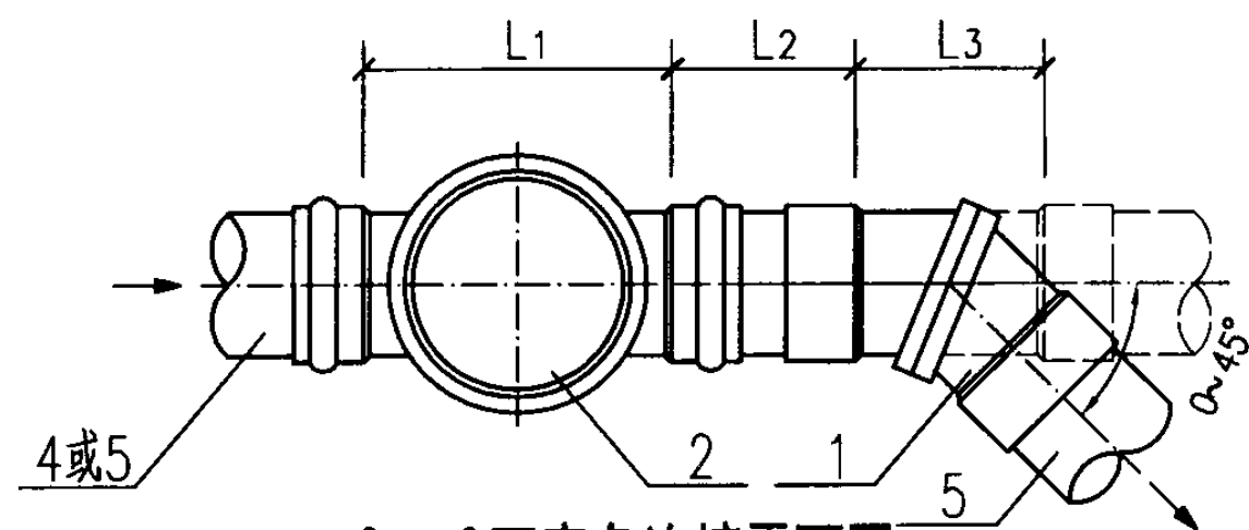
0°~45° 可变角连接平面图
