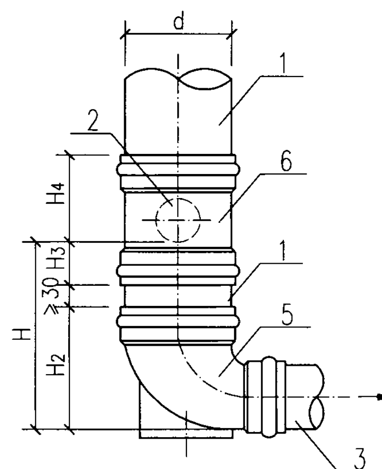
B型立面图
