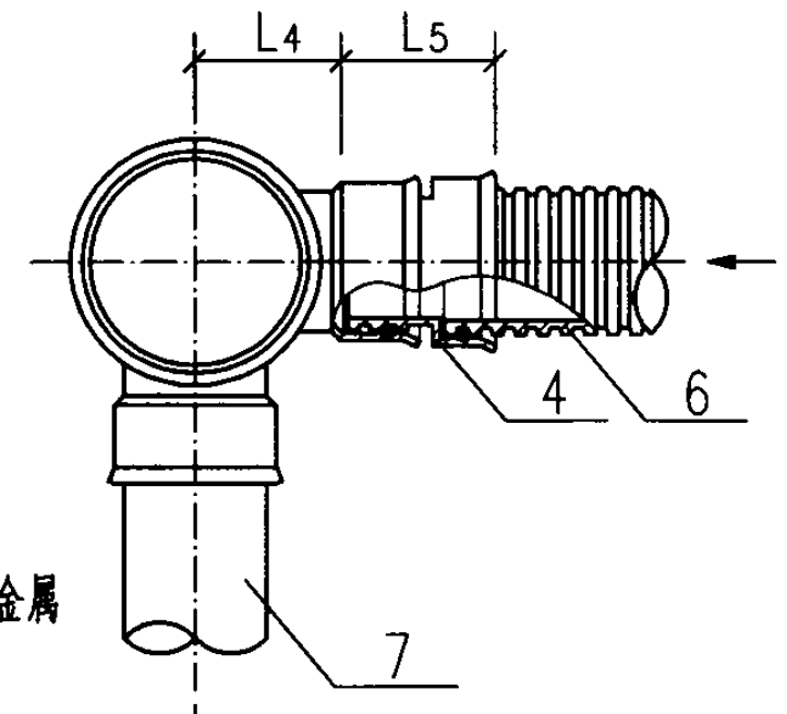
B型平面图
