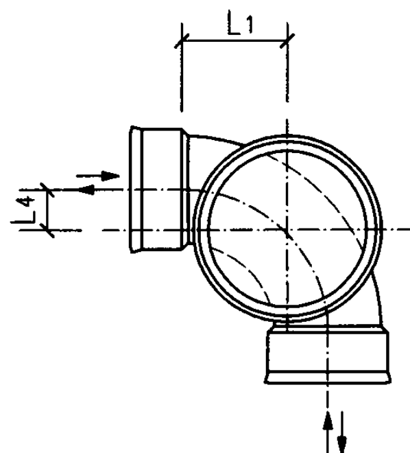
a型平面图
