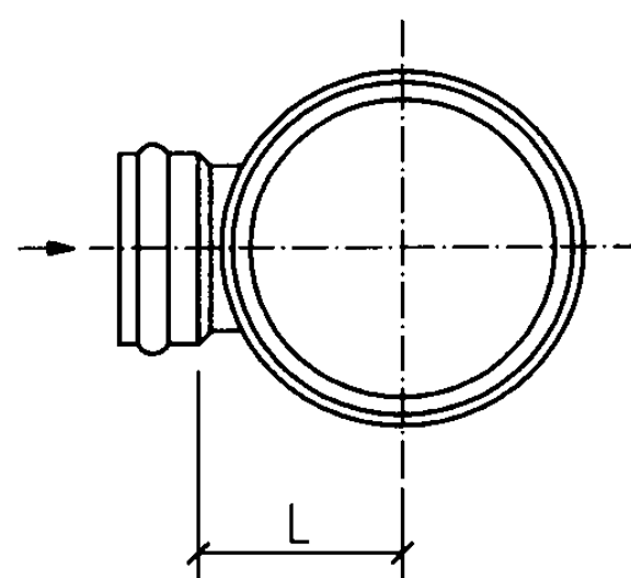
a型平面图 (一)
