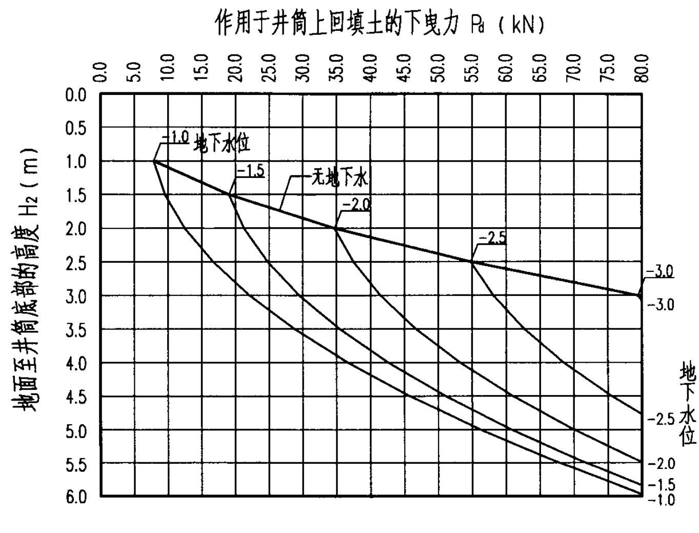
de450井筒回填土下曳力图(软土土质)
