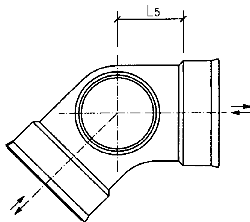
d、e型平面图
