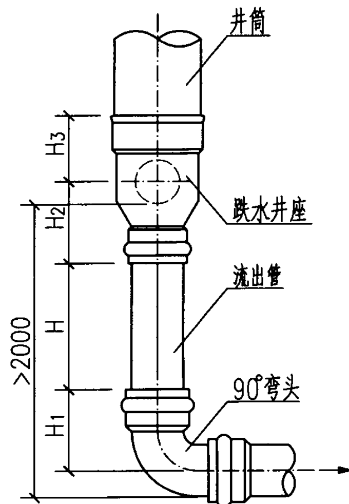
立面图
