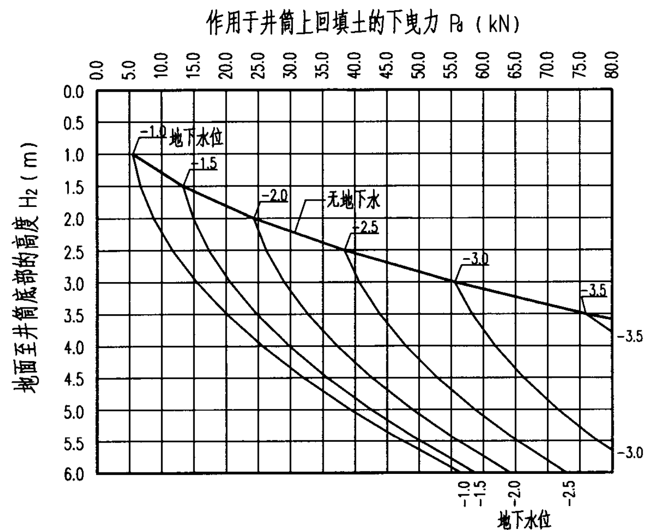
de315井筒回填土下曳力图(软土土质)
