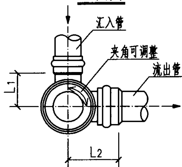
跌水井平面图
