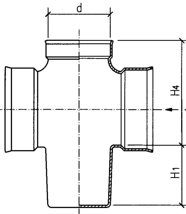
c型立、剖面图
