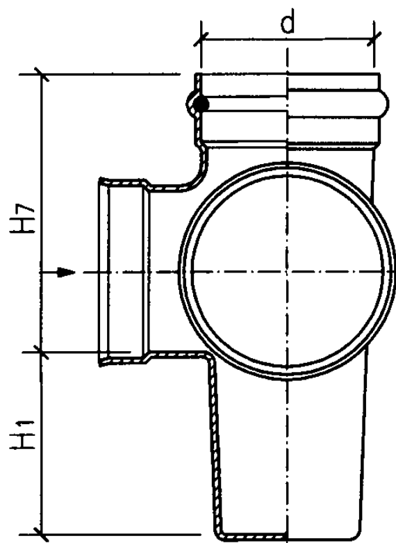
f型立、剖面图
