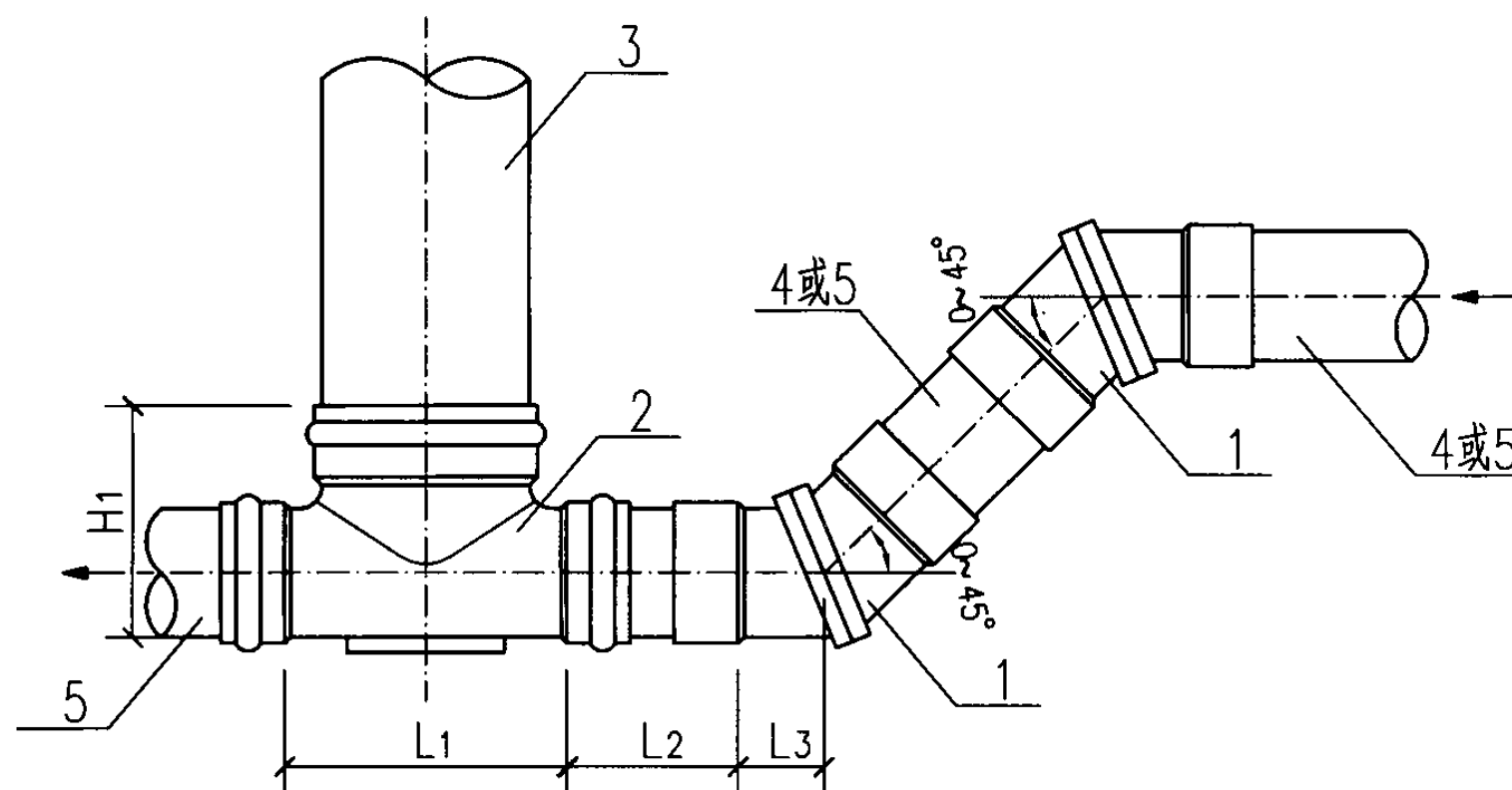
可变角变坡连接立面图
