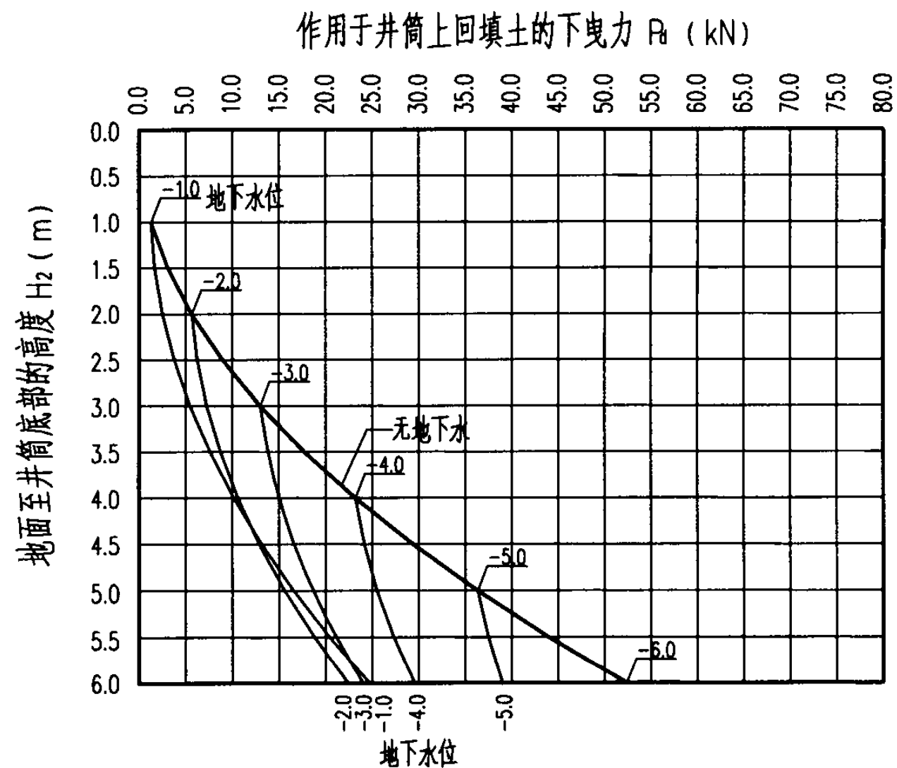
de315井筒回填土下曳力图(砂土土质)
