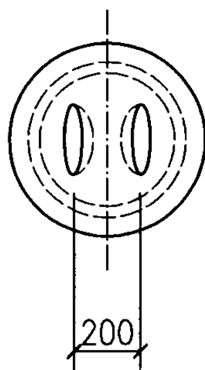
内盖平面图
