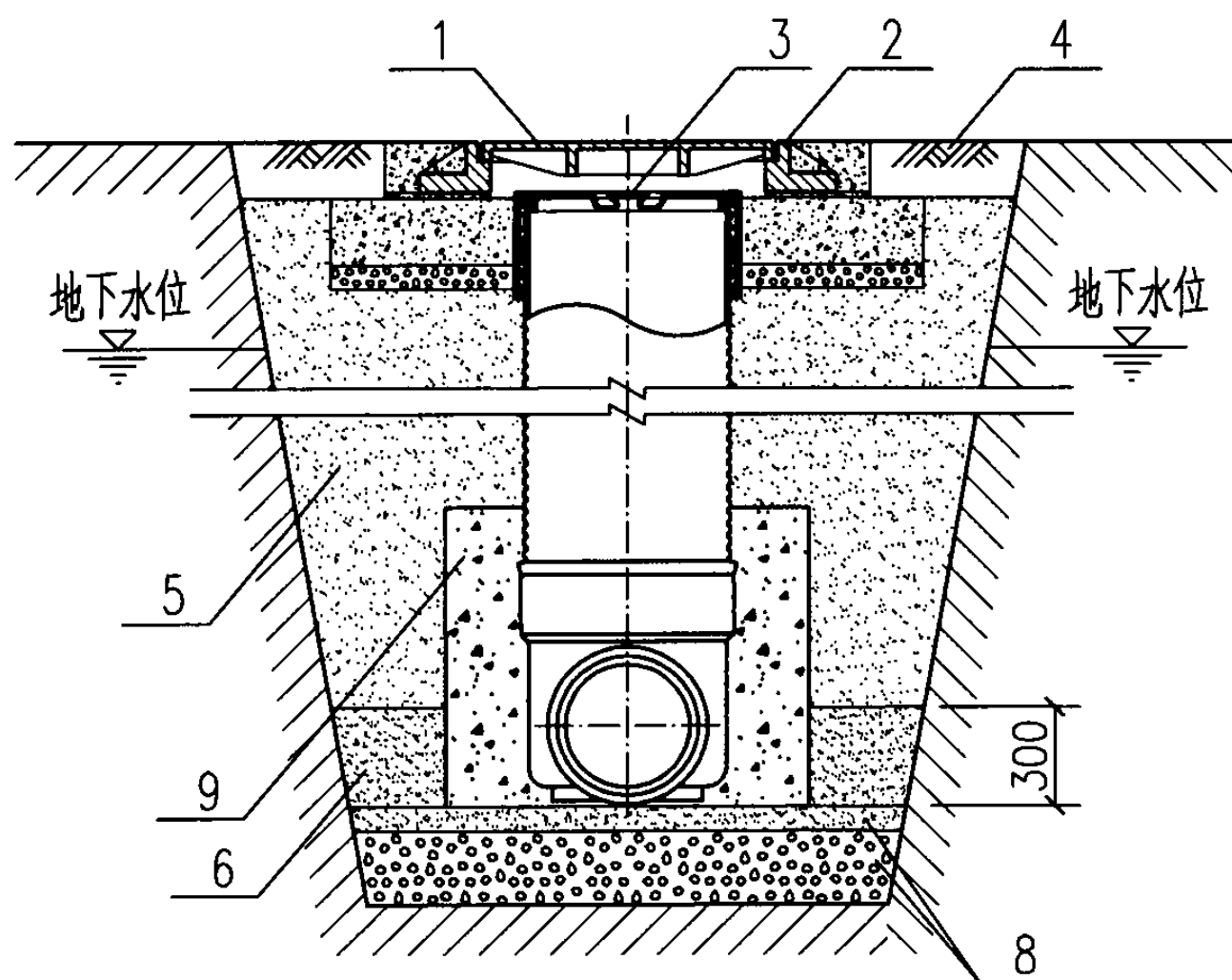
抗浮处理回填
