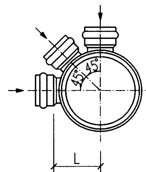
a型平面图 (三)
