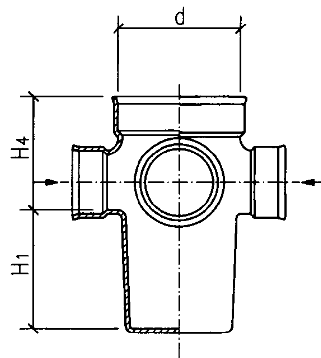
c型立、剖面图
