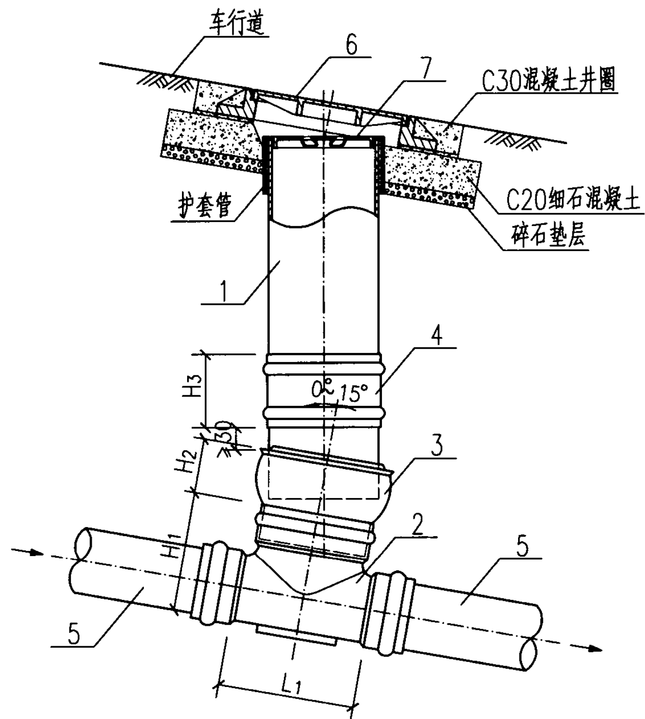
倾斜地面安装立、剖面图
