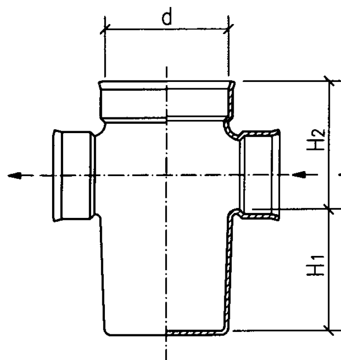
a型立、剖面图
