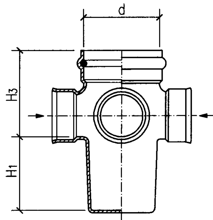
b型立、剖面图
