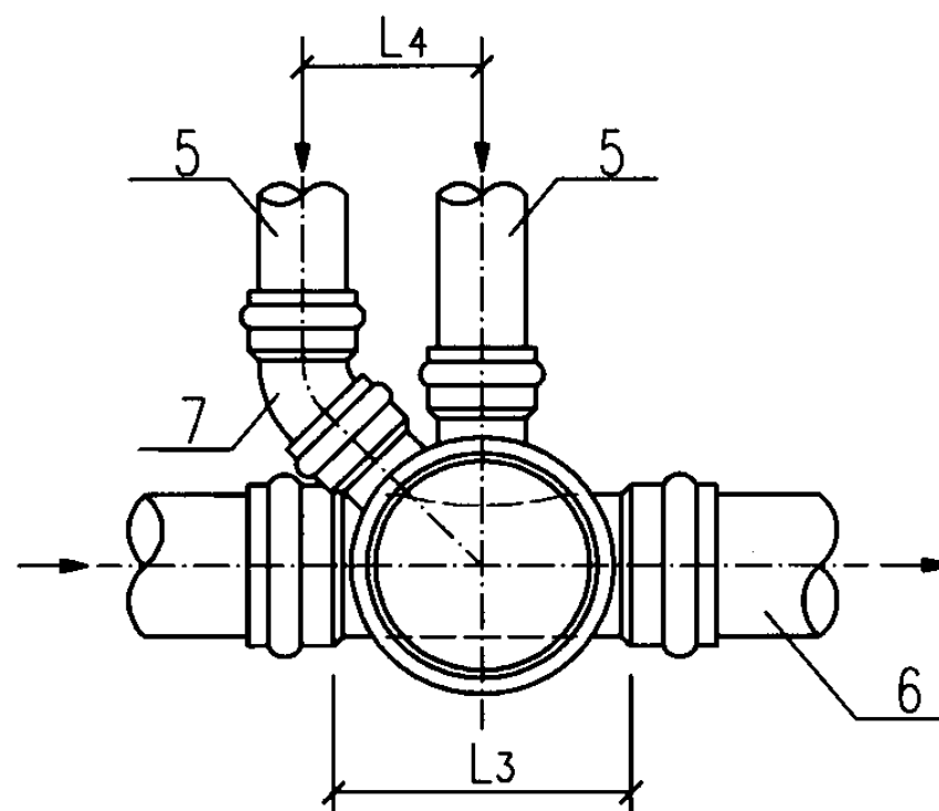
B型平面图
