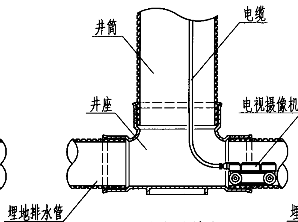
电视摄像检查
