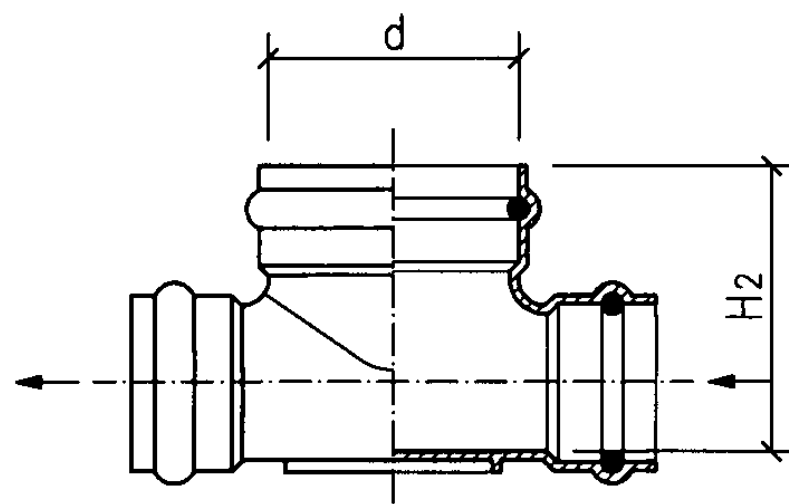
b型立、剖面图
