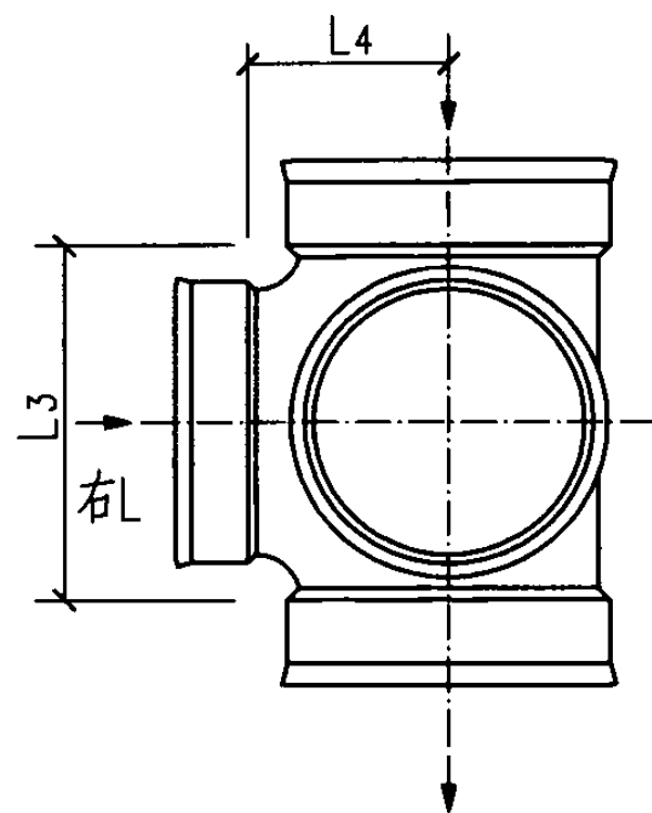
f型平面图
