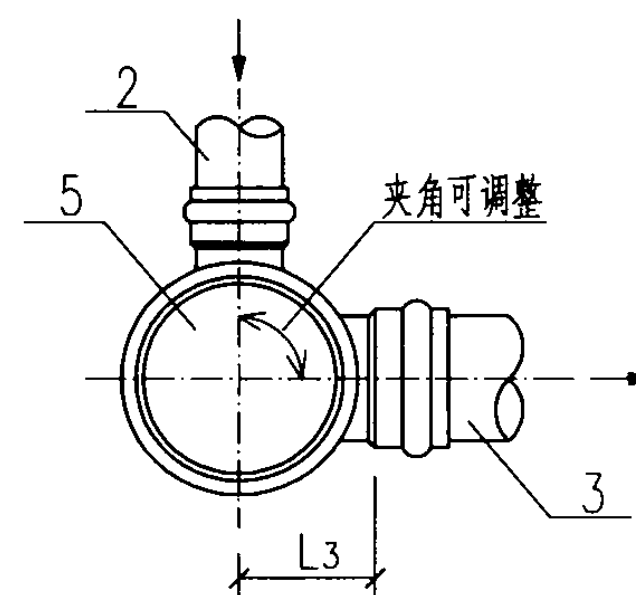
B型平面图
