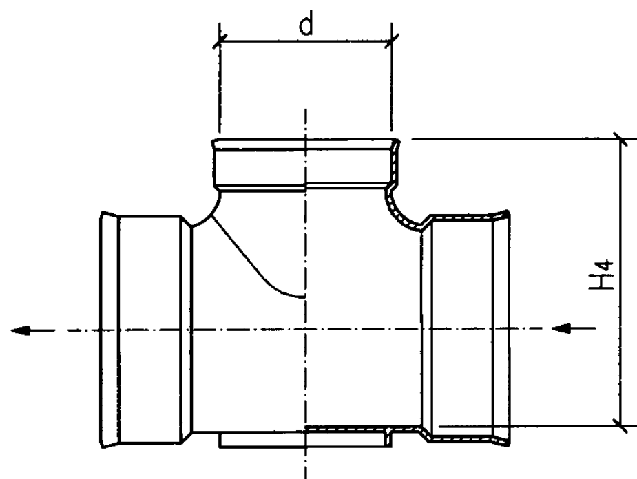
d型立、剖面图
