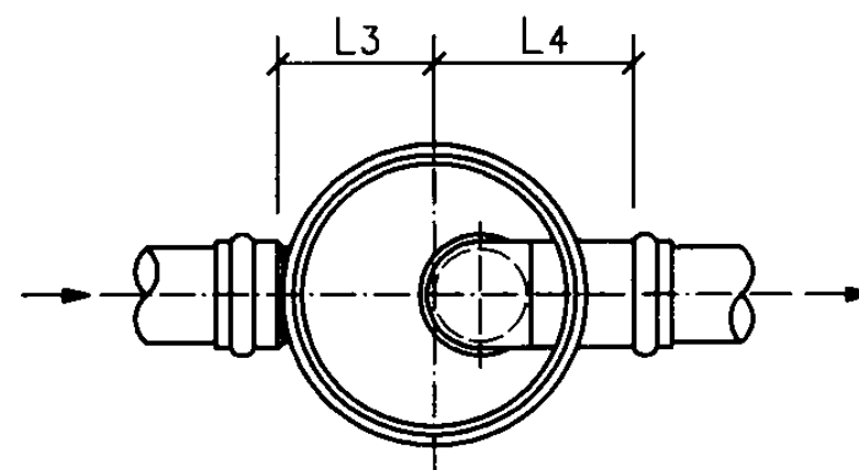
水封井平面图
