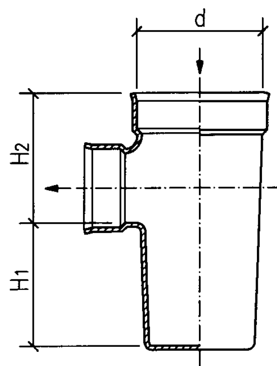
a型立、剖面图
